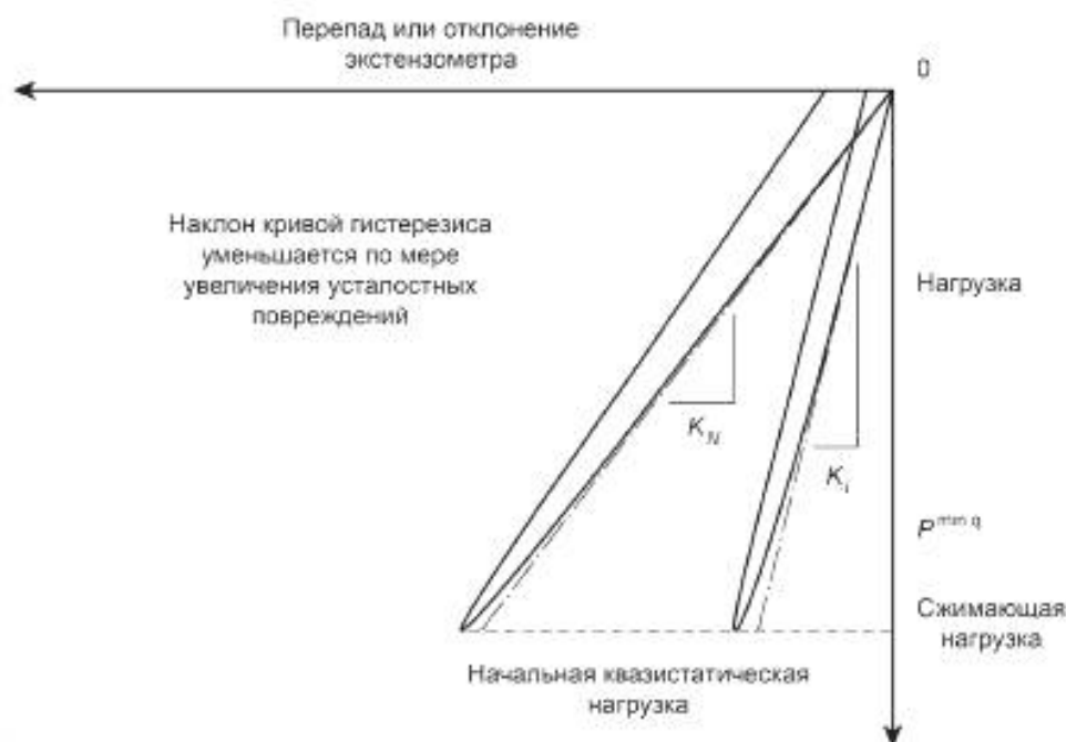
Рисунок 2 — Типичные графики зависимости сжимающего усилия от отклонения с изображением формы и параметров кривой гистерезиса
