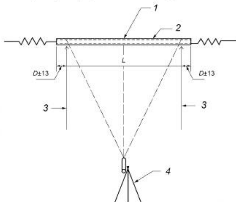
Рисунок 2 — Схема установки образца
