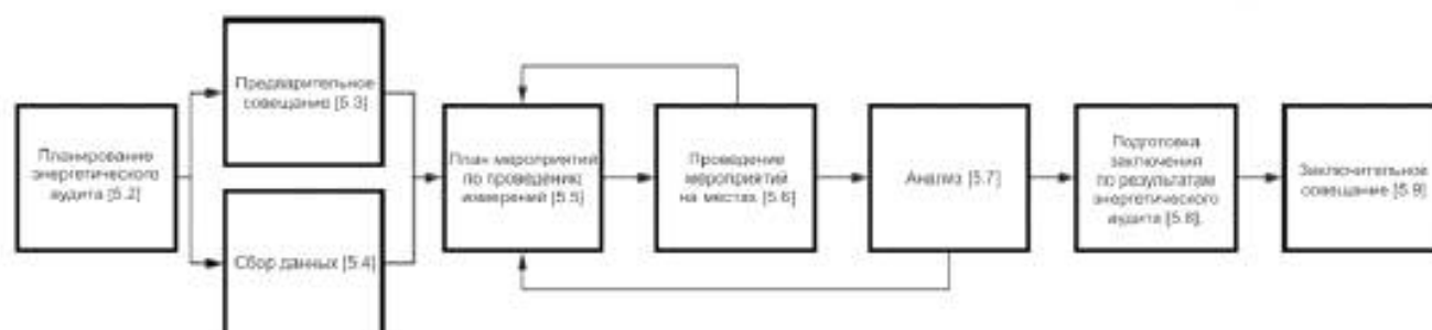
Рисунок 1 — Блок-схема процесса энергетического аудита
