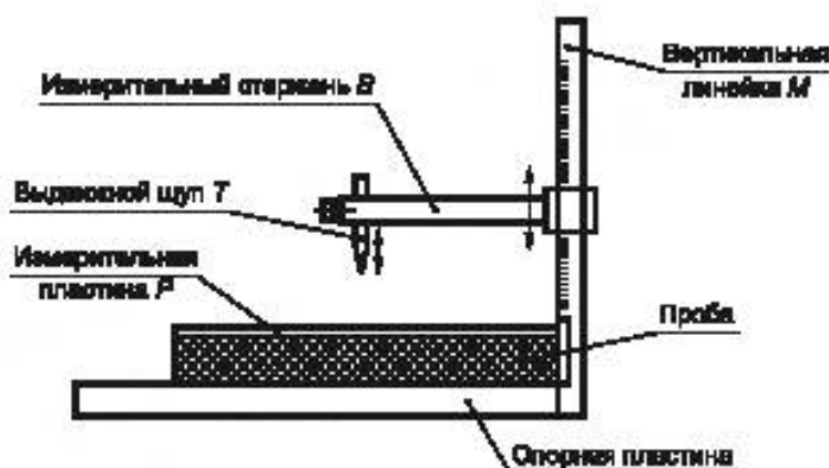
Рисунок 2 — Испытательное устройство для объемных нетканых полотен с толщиной более 20 мм
