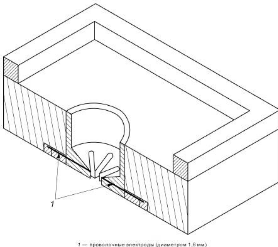
Рисунок 2 — Сечение пластины для проникания по центральной линии полости диаметром 25 мм
