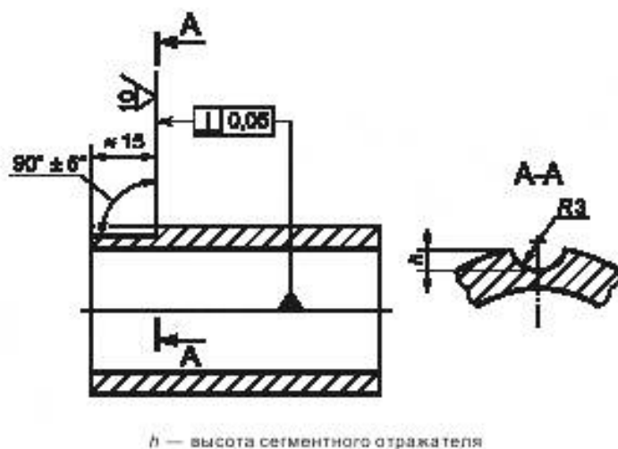
Рисунок 10 — Искусственный отражатель типа сегментного отражателя (наружная поверхность образца)
