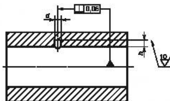
Рисунок 13 — Искусственный отражатель типа прямоугольный паз
