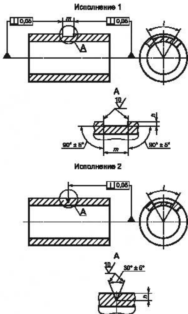
Рисунок 8 — Искусственный отражатель типа риски (наружная поверхность образца)
