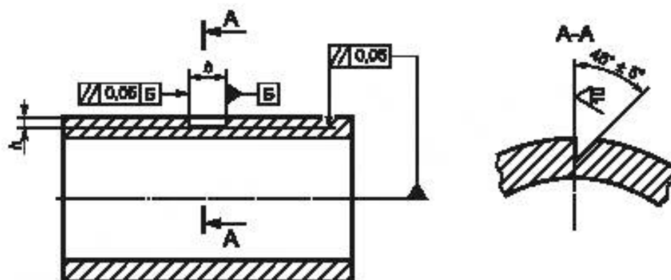
Рисунок 6 — Искусственный отражатель типа зарубки (наружная поверхность образца)
