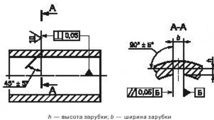
Рисунок 11 — Искусственный отражатель типа зарубки (внутренняя поверхность образца)
