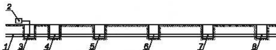
1 — трубопровод; 2 — виброакустический прибор; 3—8 — места установки микрофонов
