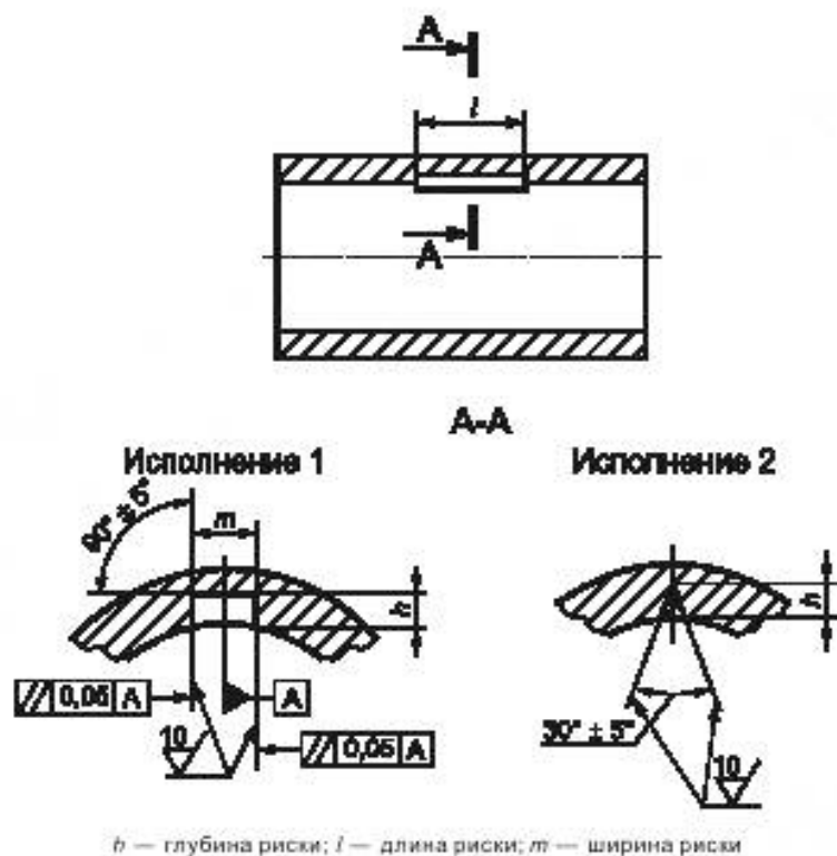
Рисунок 1 — Искусственный отражатель типа риски (внутренняя поверхность образца)
