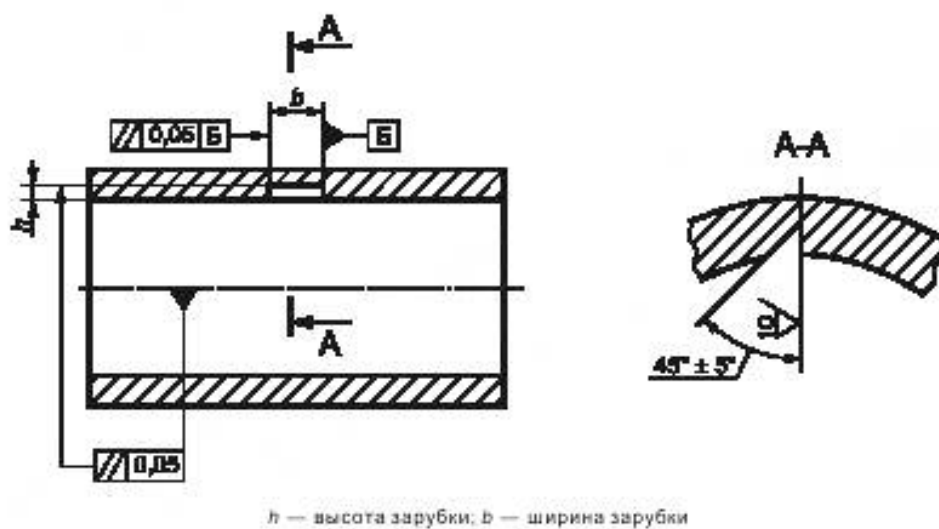
Рисунок 5 — Искусственный отражатель типа зарубки (внутренняя поверхность образца)
