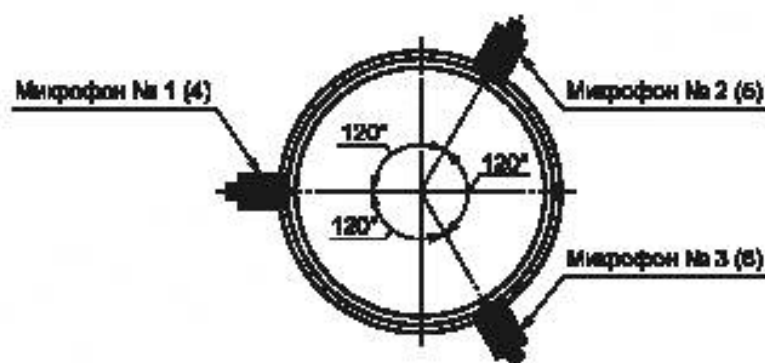
Рисунок 16 — Схема установки микрофонов на участок трубопровода
