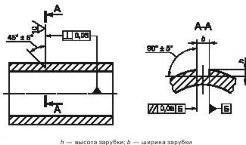
Рисунок 12 — Искусственный отражатель типа зарубки (наружная поверхность образца)
