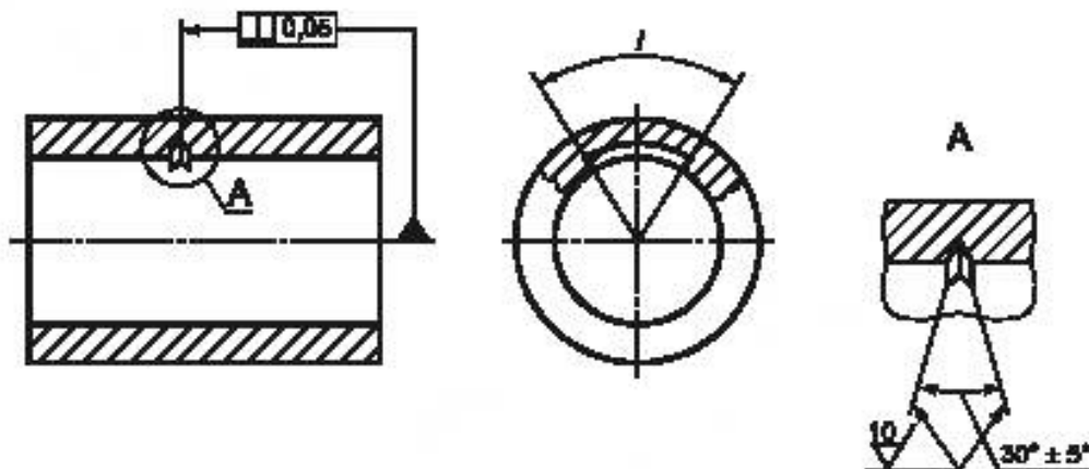
Рисунок 7 — Искусственный отражатель типа риски (внутренняя поверхность образца)
