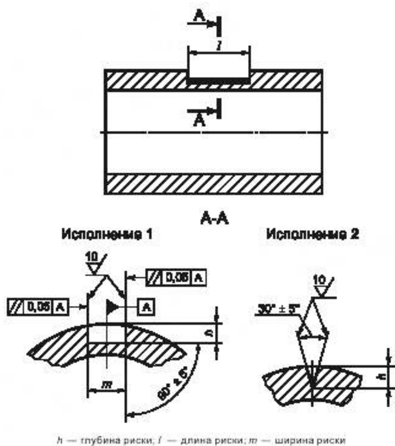
Рисунок 2 — Искусственный отражатель типа риски (наружная поверхность образца)
