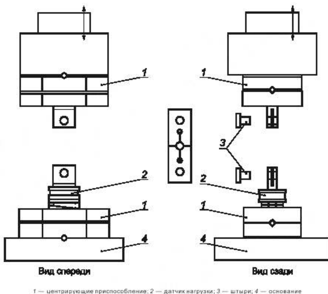
Рисунок 2 — Общая схема машины для испытания для определения предела прочности при растяжении
