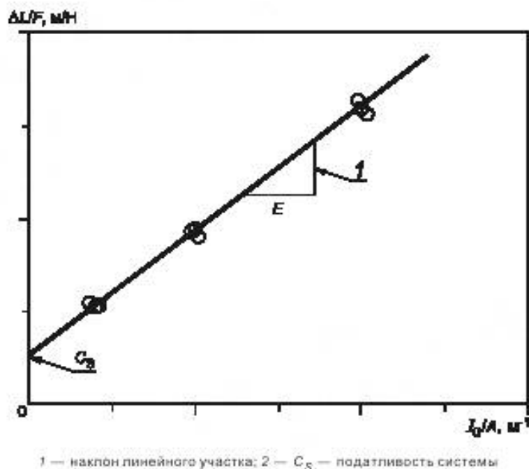
Рисунок 6 — Пример графика для определения податливости системы
