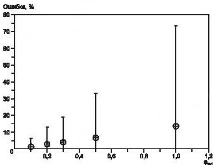
Рисунок X1.3 — Погрешность при определении предела прочности при растяжении волокна в зависимости от переменной диаметра волокна ( \varphi_{sd} ) по его длине
