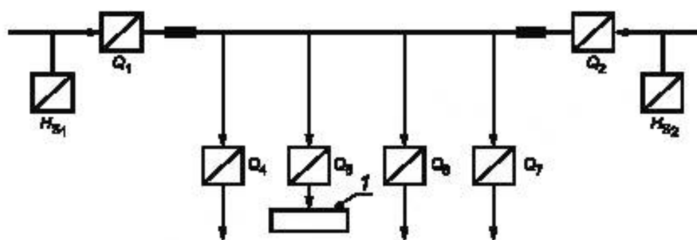
Q_1, Q_4, Q_5, Q_6 и Q_7 — пункты приема-передачи; 1 — промышленный потребитель
