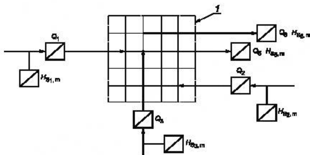
1 — модель сети газопроводов; Q_1, Q_2, Q_3, Q_5, Q_6 — пункты приема-передачи
