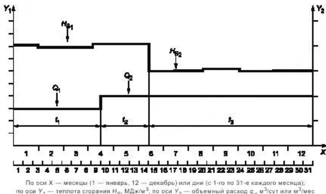
Рисунок В.2 — Определение энергии с периодом в один год или один месяц с двумя разными теплотами сгорания
