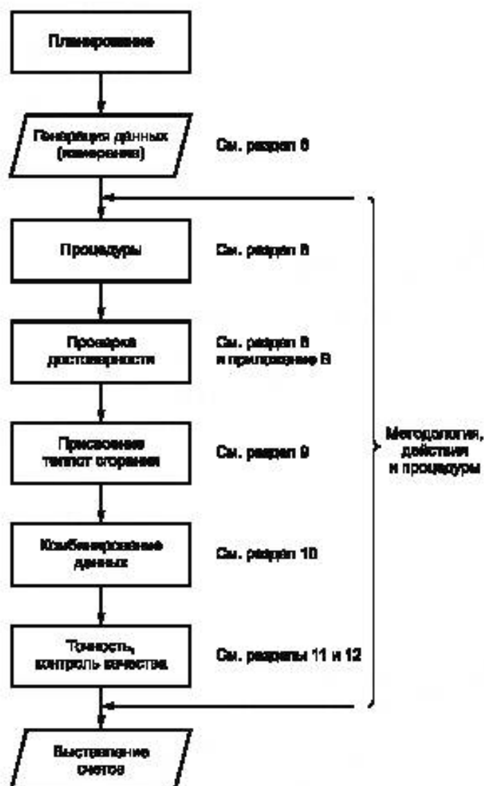
Рисунок 9 — Схема косвенного метода определения энергии
