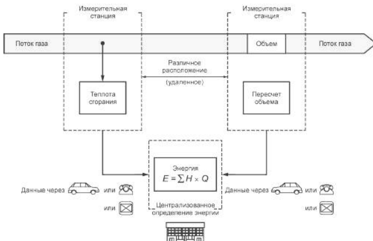
Рисунок 8 — Удаленное измерение теплоты сгорания (пример)
