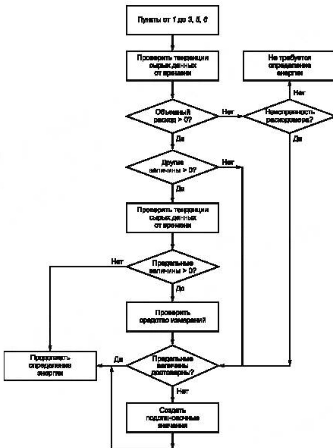
Рисунок 11 — Схема алгоритма проверки достоверности данных
