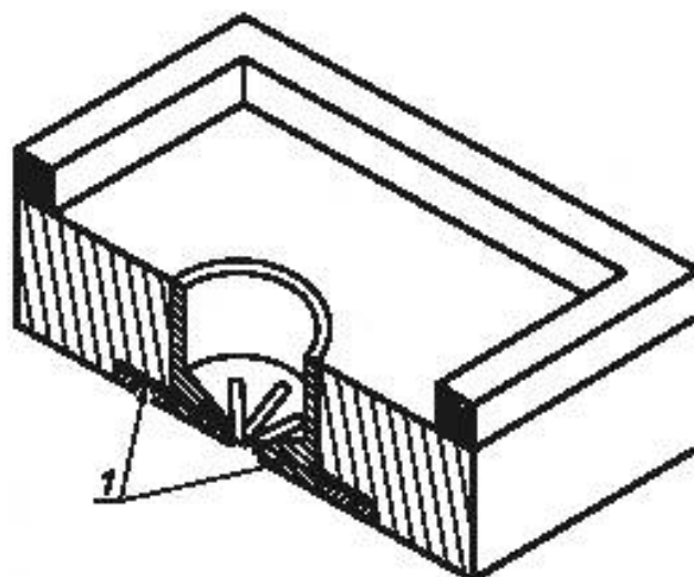
1 — проволочные электроды (диаметром 1,6 мм)
