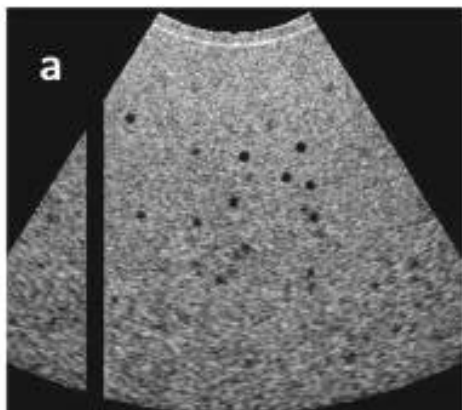
а Обрезанное изображение из рисунка В.1 с удаленной вертикальной линией, сформированной слабыми рассеянными эхосигналами от поверхности плоской алюминиевой пластины
