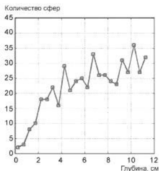
Рисунок J.1 — Результаты для сканера системы A и датчика 7CF2 3D (качающаяся конвексная решетка) с фокусным расстоянием 4 см, работающего на частоте 4,5 МГц в режиме 2D-сканирования
