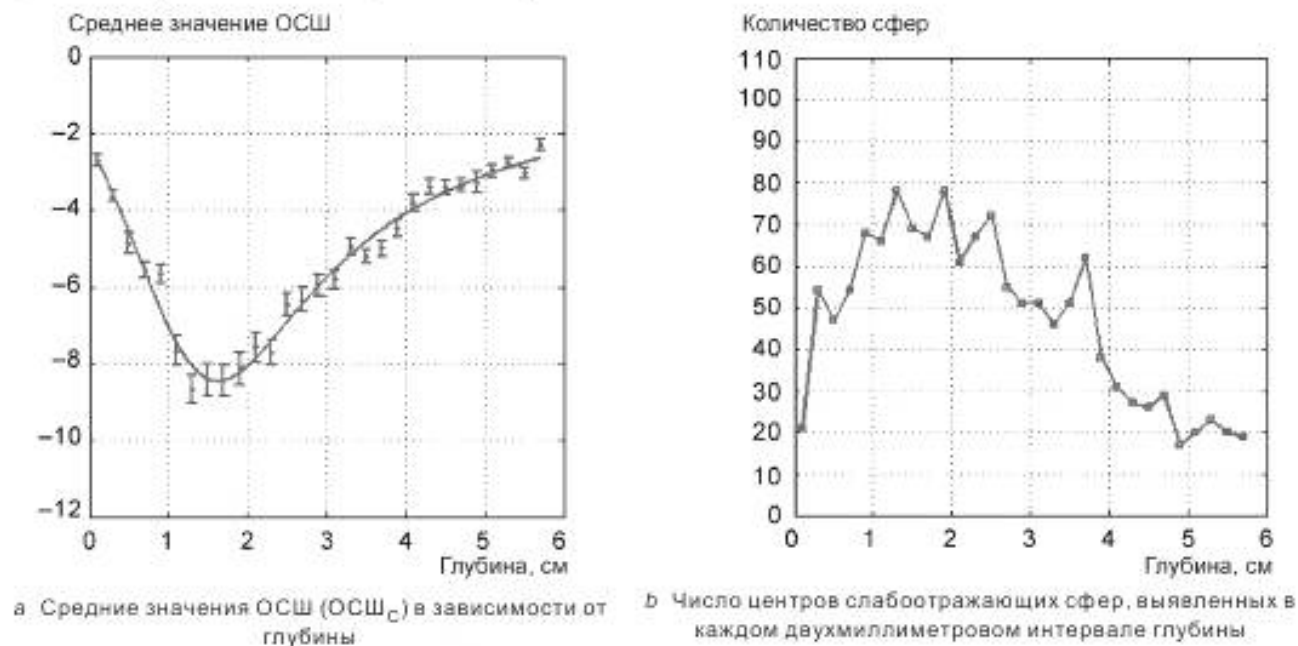
Рисунок С.13 — Результаты, полученные при использовании всех 200 изображений из набора, соответствующего набору на рисунке С.12
