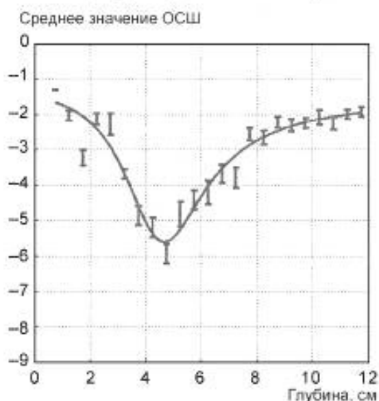
Рисунок J.2 — Результаты для сканера системы B и датчика 4DC7-3 3D (конвексная решетка) с фокусным расстоянием 4 см, работающего на частоте 4 МГц в режиме 2D-сканирования. Угол сектора и все другие настройки панели управления имитировали настройки системы A (рисунок J.1)
