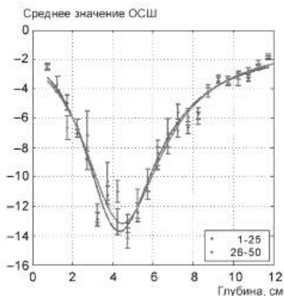
а Средние значения ОСШ (ОСШ с ) в зависимости от глубины в соответствии с двумя независимыми наборами из 25 изображений, относящиеся к рисункам В.1 и В.2
