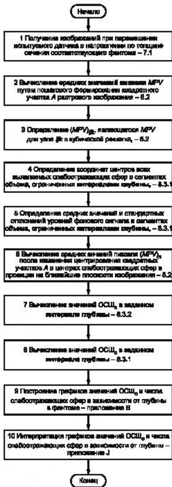
Рисунок 1 — Структурная схема
