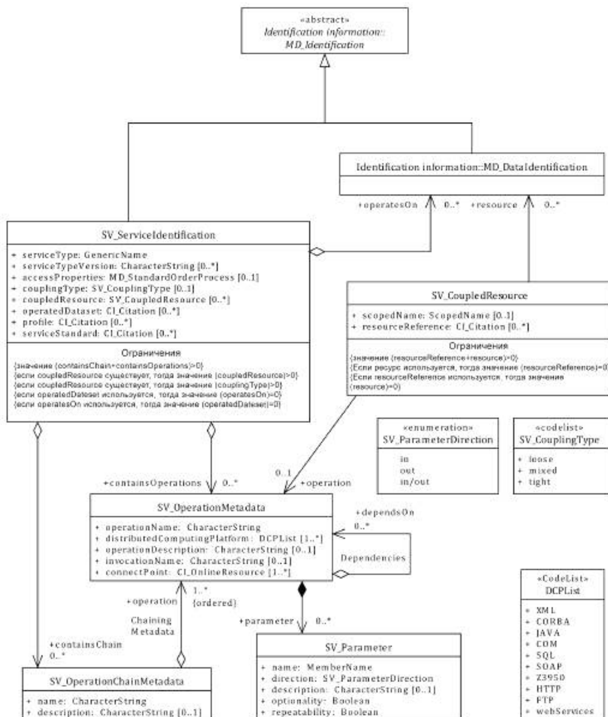
Рисунок 18 — Классы информации о метаданных на сервисы
