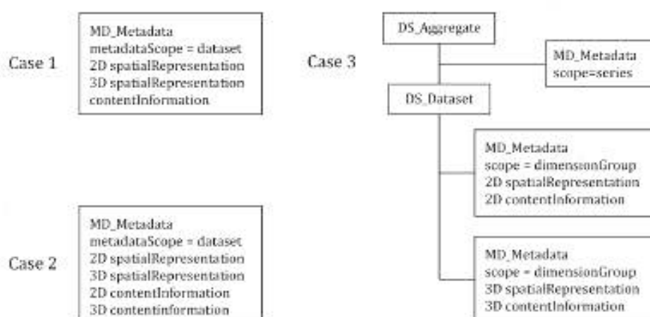
Рисунок E.1 — Области применения метаданных
