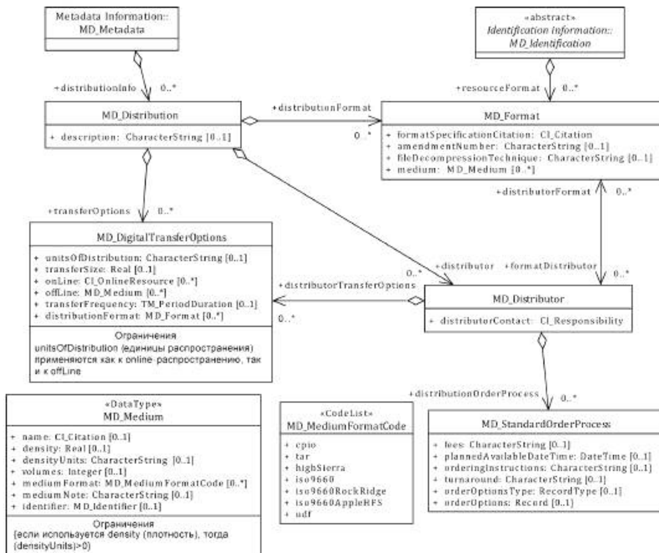
Рисунок 15 — Классы информации о распространении
