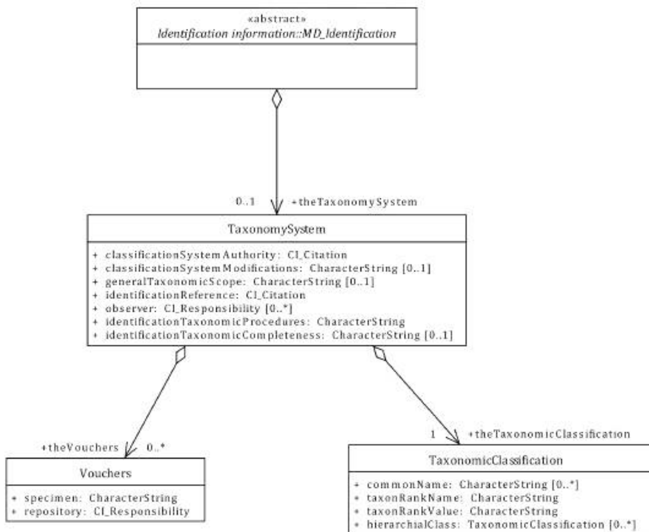
Рисунок D.1 — Пример расширенных данных
