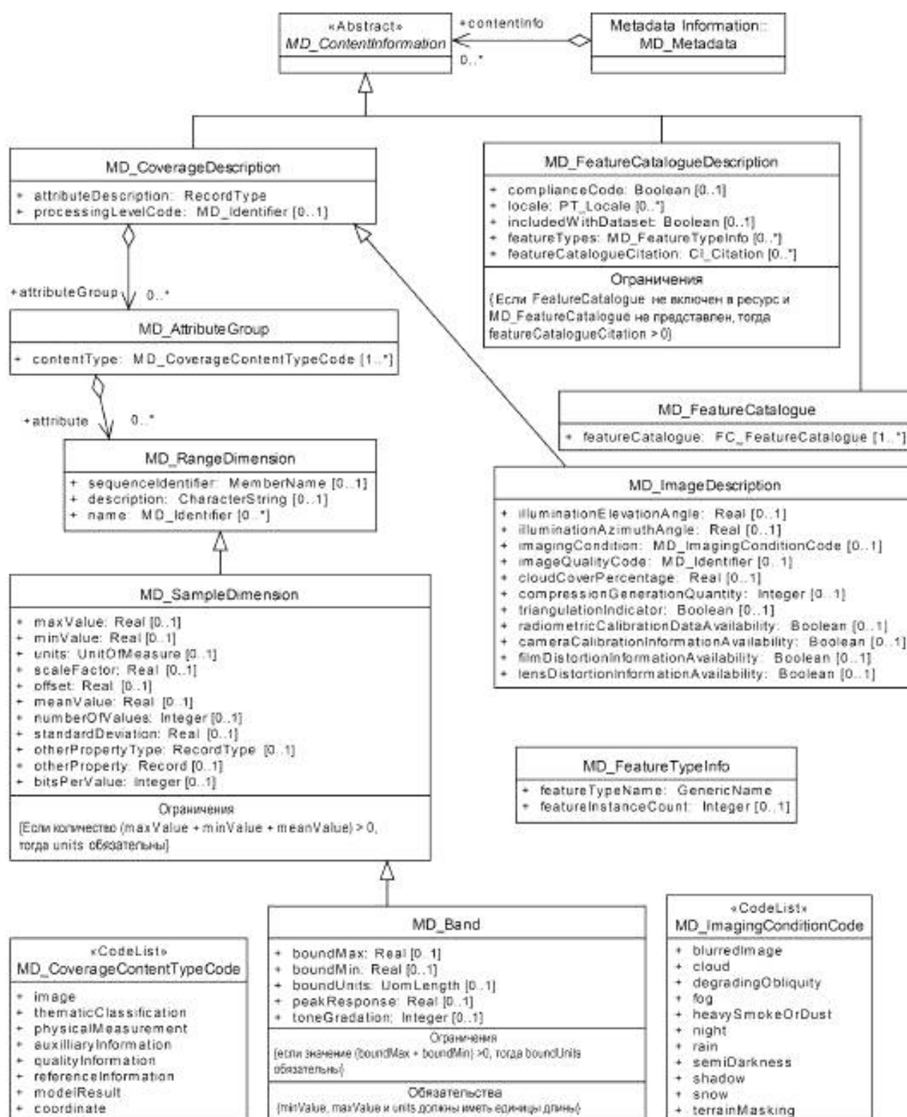
Рисунок 13 — Классы информации о содержании
