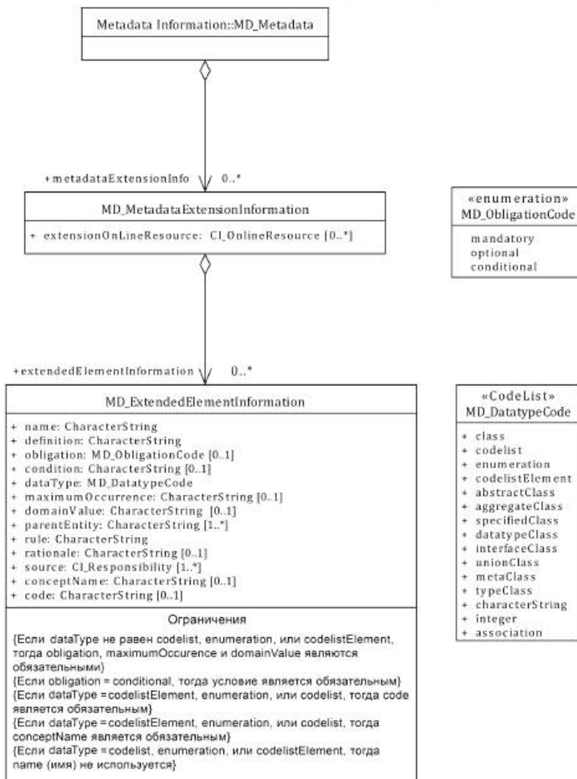
Рисунок 16 — Классы Информации о расширении метаданных
