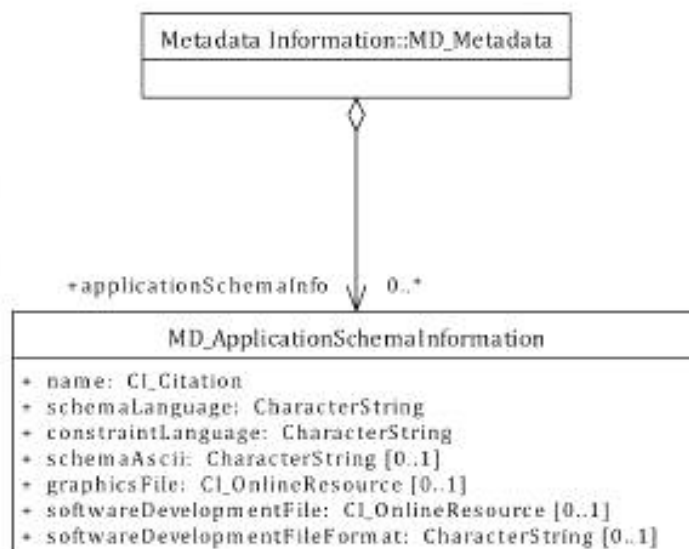
Рисунок 17 — Класс информации о прикладной схеме
