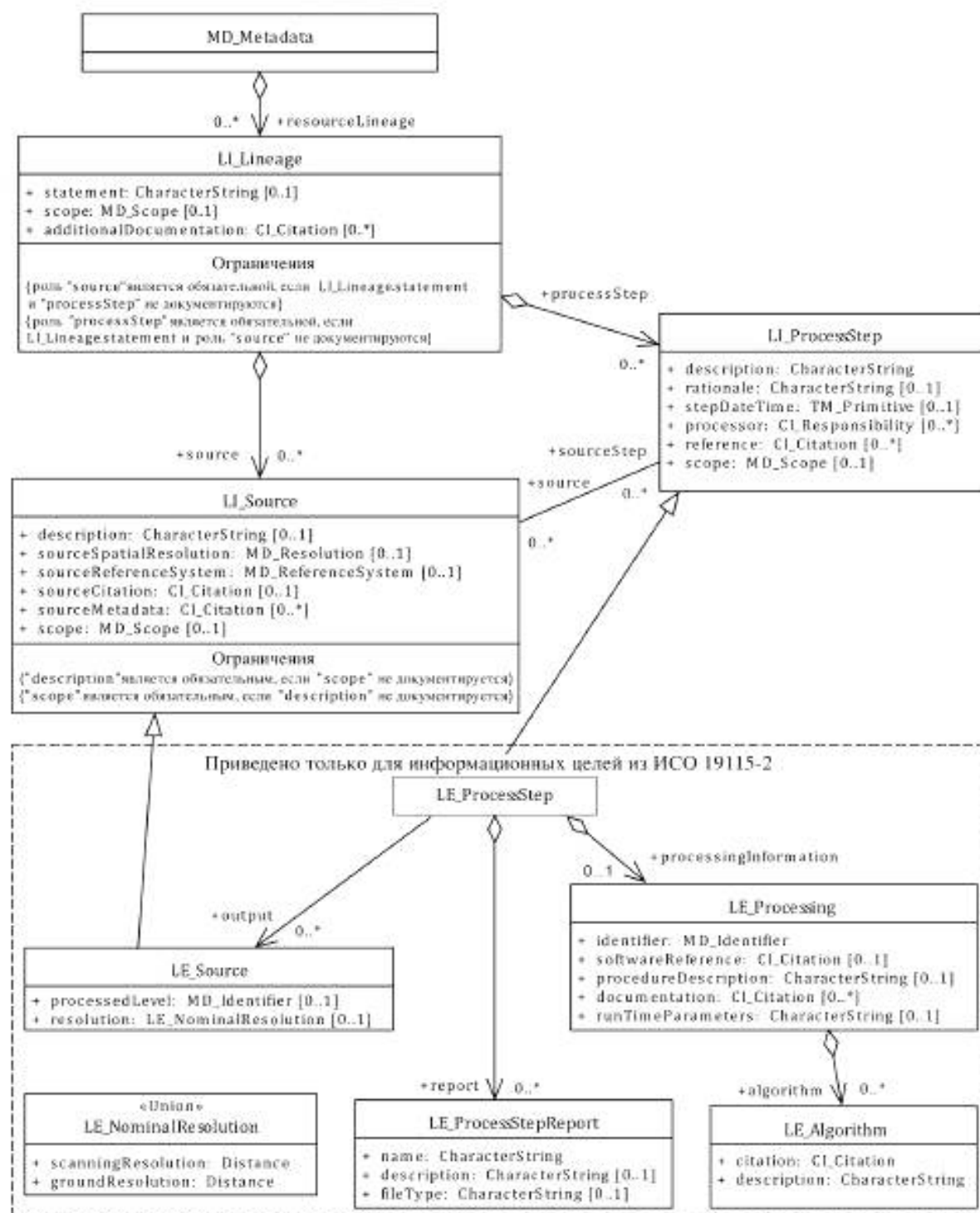
Рисунок 9 — Классы информации о происхождении
