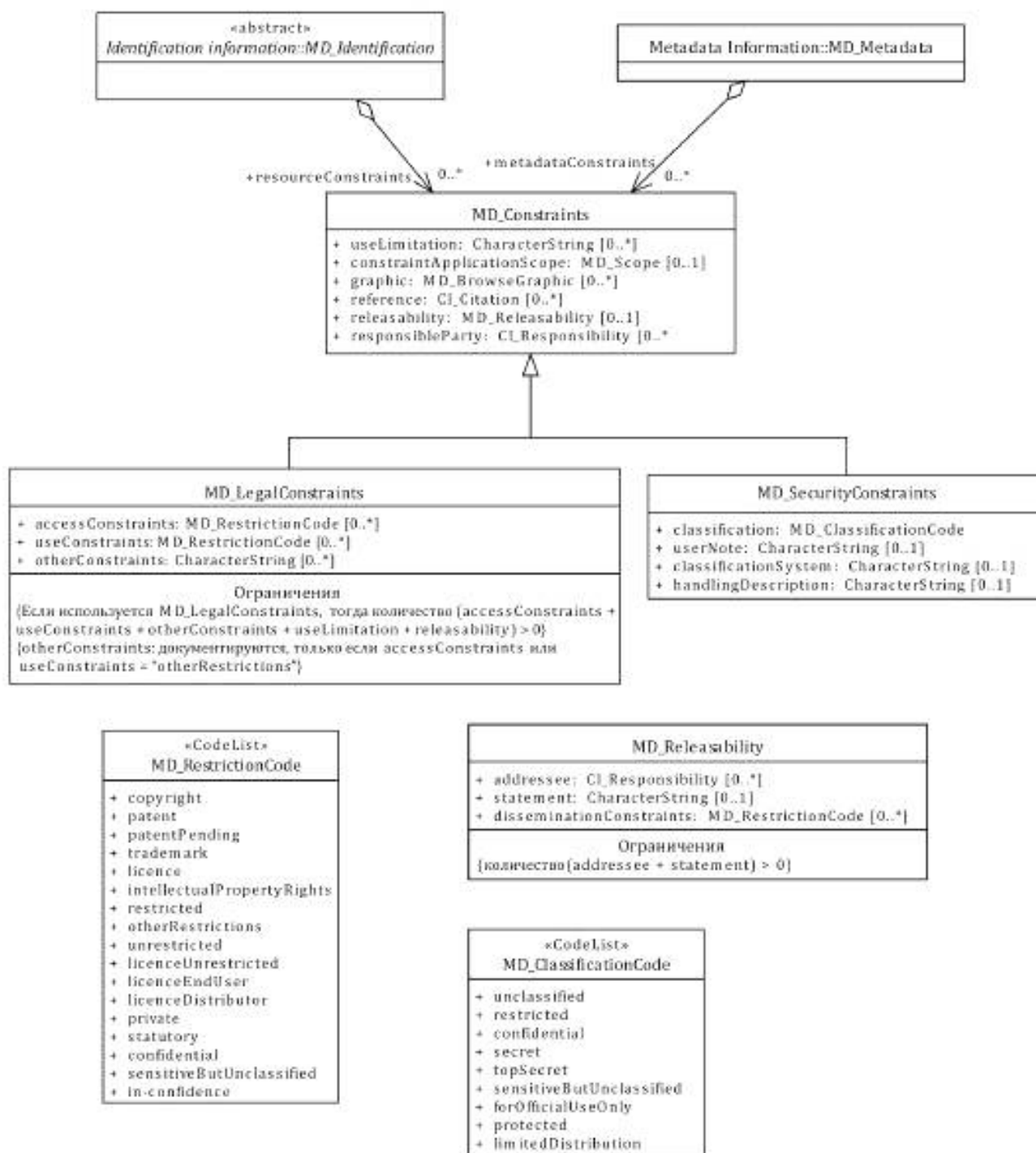
Рисунок 8 — Классы информации об ограничениях
