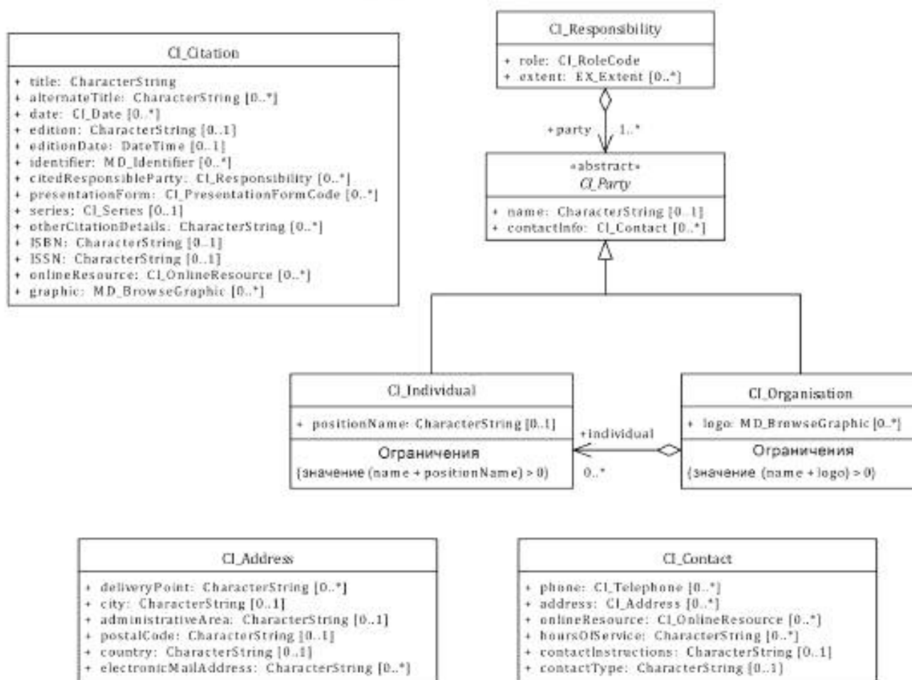
Рисунок 20 — Классы информации о ссылках и ответственном субъекте
