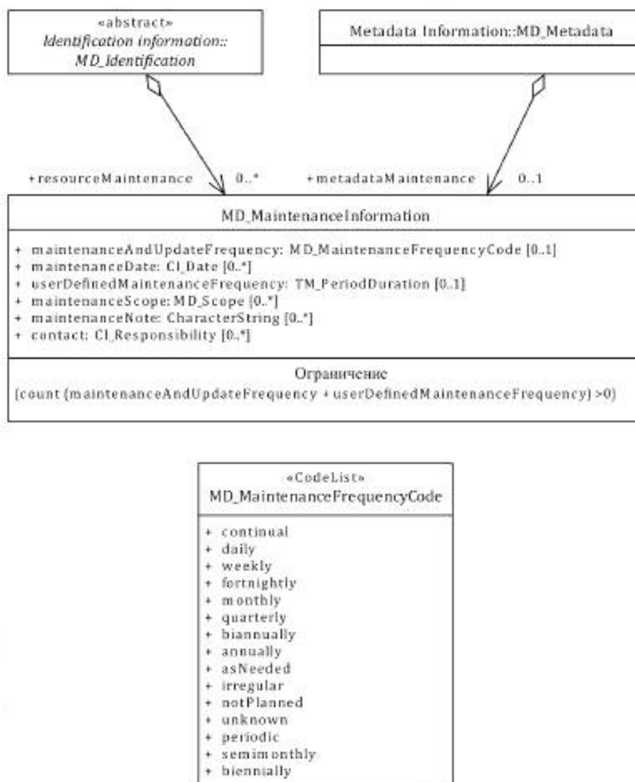
Рисунок 10 — Классы информации по ведению данных
