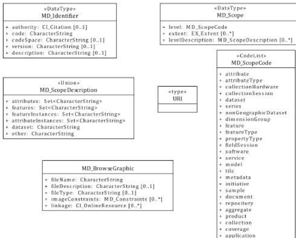
Рисунок 22 — Общеиспользуемые классы
