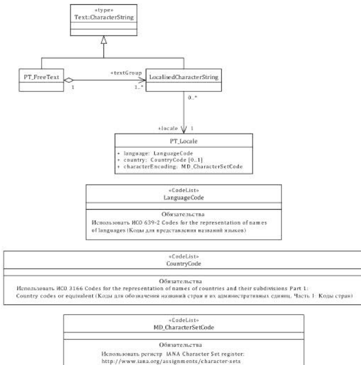
Рисунок 23 — Схема PT_Locale
