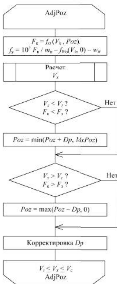
Рисунок А.3 — Схема алгоритма уточнения позиции управления силой тяги
