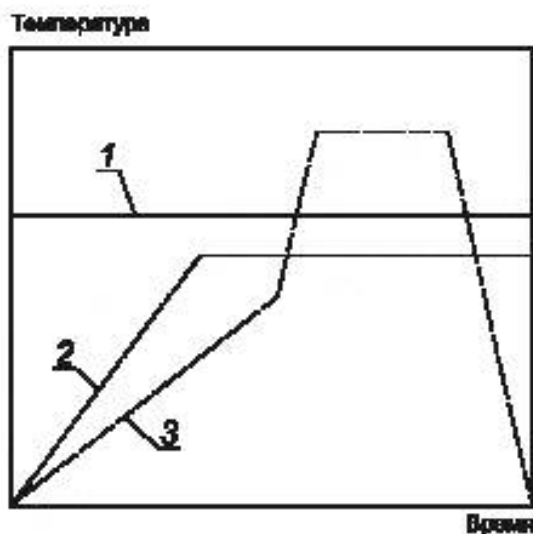
1 — кривая изотермического отверждения; 2 — схема изменения температуры; 3 — имитация технологического процесса
