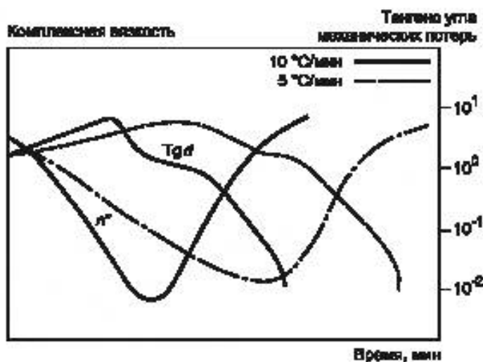
Рисунок 2 — Примеры кривых отверждения при различных температурных градиентах
