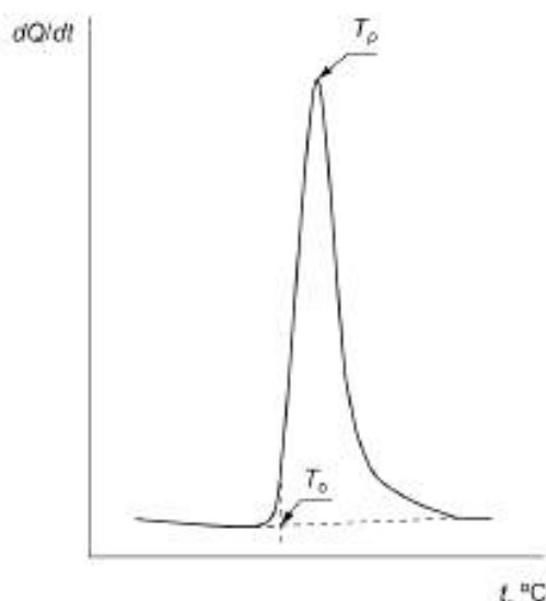
Рисунок 1 — Типовая кривая экзотермического отверждения
