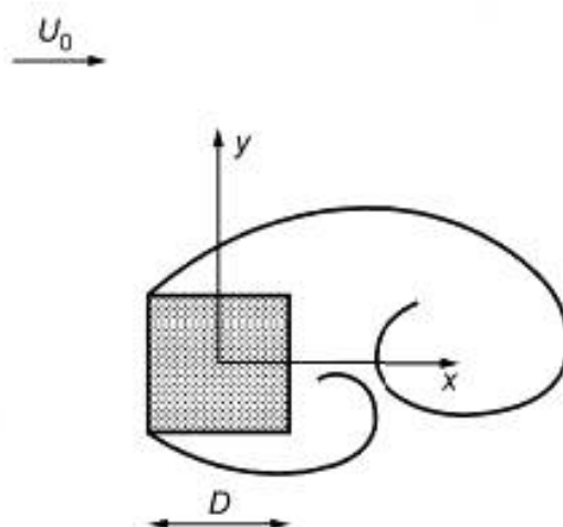
Рисунок 54 — Турбулентная дорожка Кармана за квадратным цилиндром
