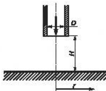
Рисунок 22 — Круглая струя, нормально падающая на плоскость
