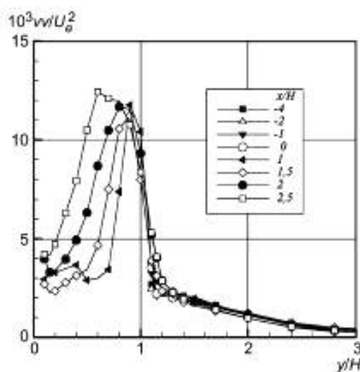
Рисунок 31 — Нормальные напряжения Рейнольдса в поперечном направлении
