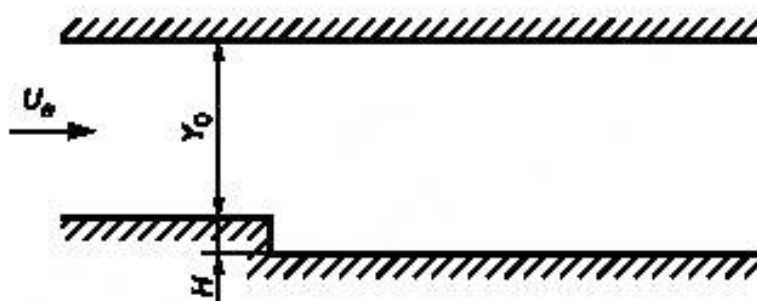
Рисунок 27 — Обтекание обратного уступа
