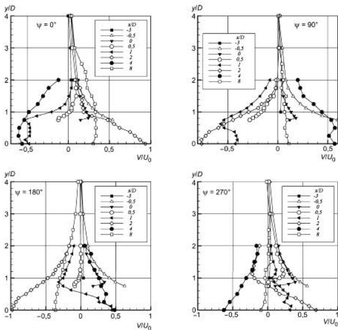
Рисунок 56 — Профили поперечной компоненты средней скорости
