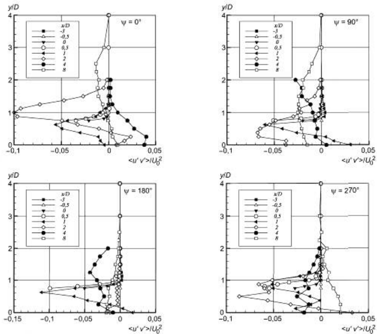
Рисунок 59 — Профили сдвиговых напряжений Рейнольдса
