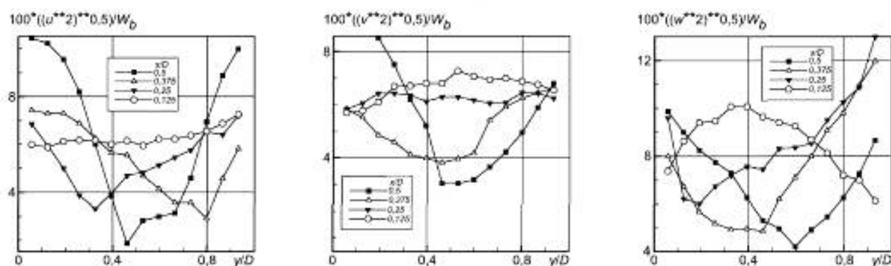
Рисунок 3 — Нормальные компоненты напряжений Рейнольдса в сечении \psi = 0
