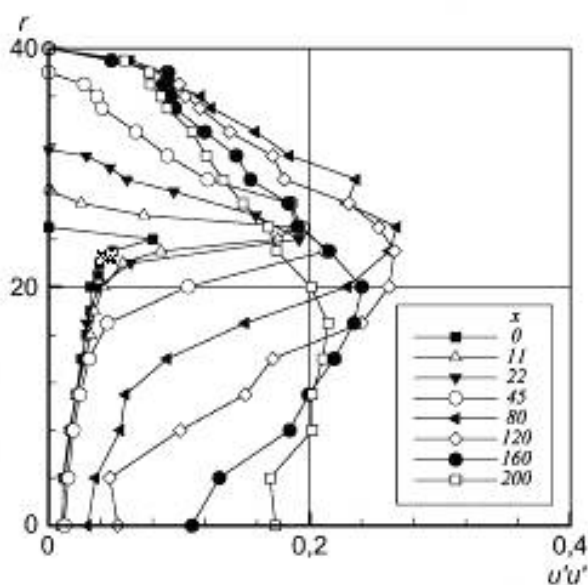
Рисунок 50 — Нормальные напряжения Рейнольдса в осевом направлении; x и r в мм, u'u' в м²/с²
