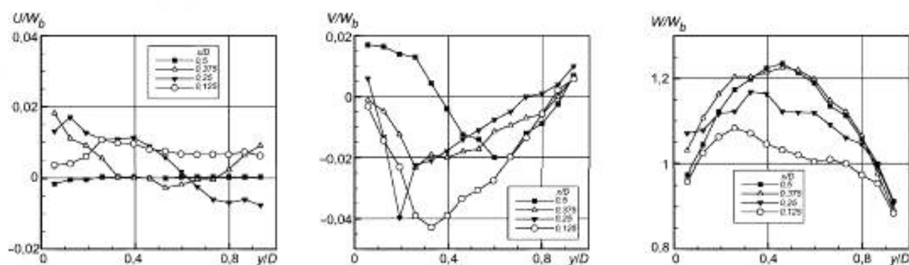
Рисунок 2 — Три компоненты скорости в сечении \psi = 0
