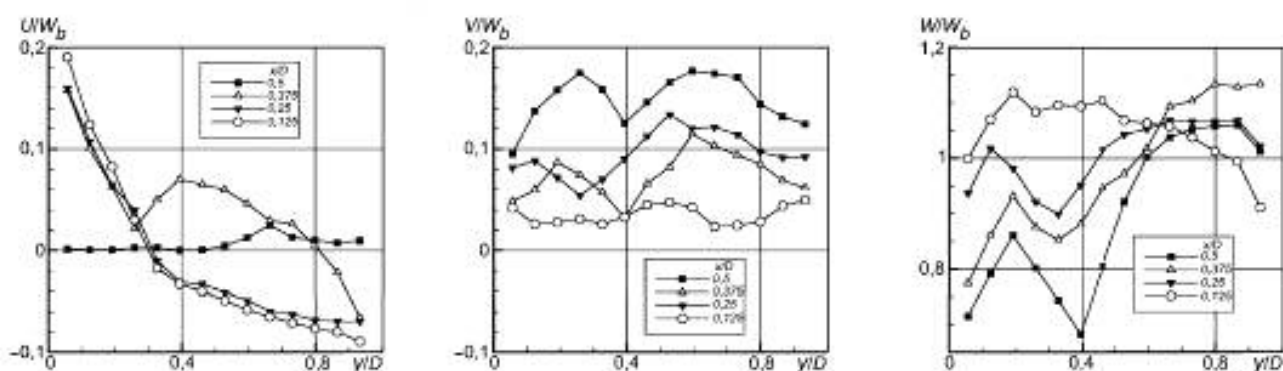
Рисунок 6 — Три компоненты скорости в сечении \psi = \pi/2
