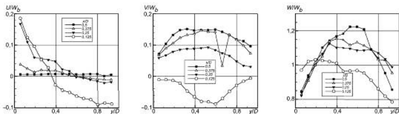
Рисунок 4 — Три компоненты скорости в сечении \psi = \pi/4
