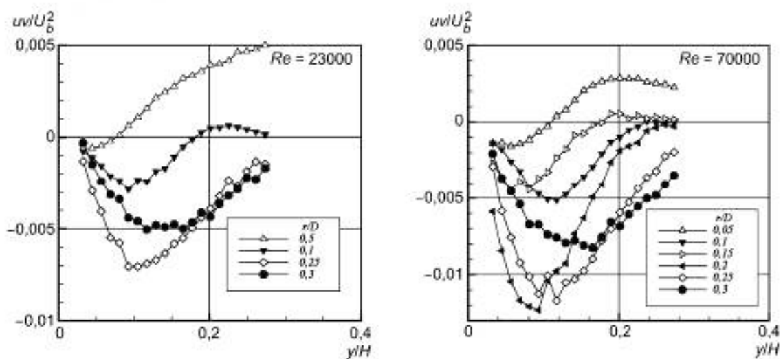
Рисунок 26 — Сдвиговые напряжения Рейнольдса
