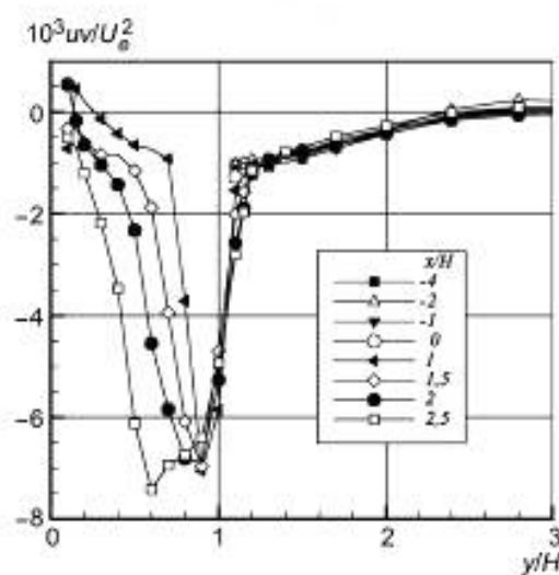
Рисунок 32 — Касательные напряжения Рейнольдса
