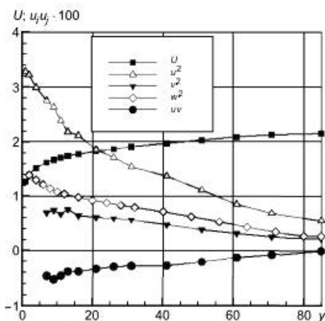
Рисунок 19 — Профиль скорости U (м/с) и профили компонент напряжений Рейнольдса u'u' (м 2 /с 2 ) в набегающем потоке. Координата y в мм
