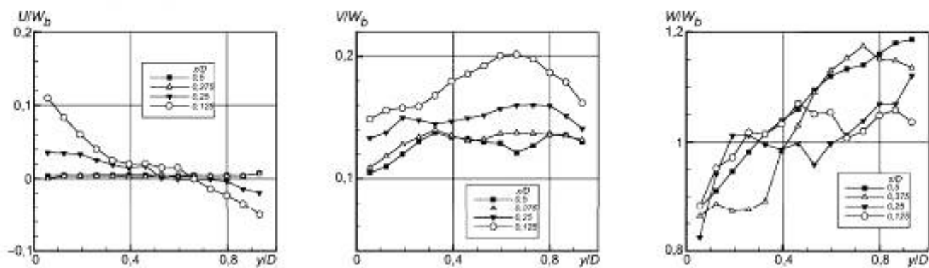
Рисунок 10 — Три компоненты скорости в сечении \psi = \pi
