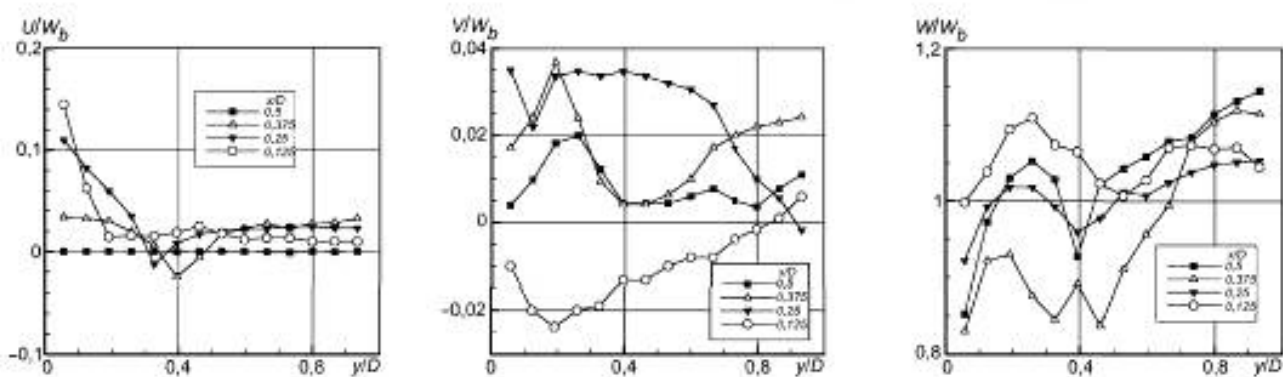
Рисунок 8 — Три компоненты скорости в сечении \psi = 3\pi/4
