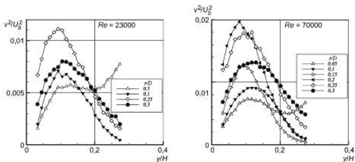
Рисунок 25 — Нормальные напряжения Рейнольдса
