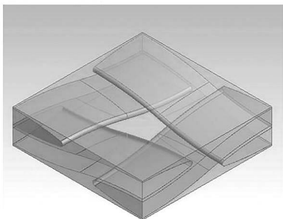
Рисунок А.8 — 1/4 ЯП ТКМ с плотной структурой плетения
