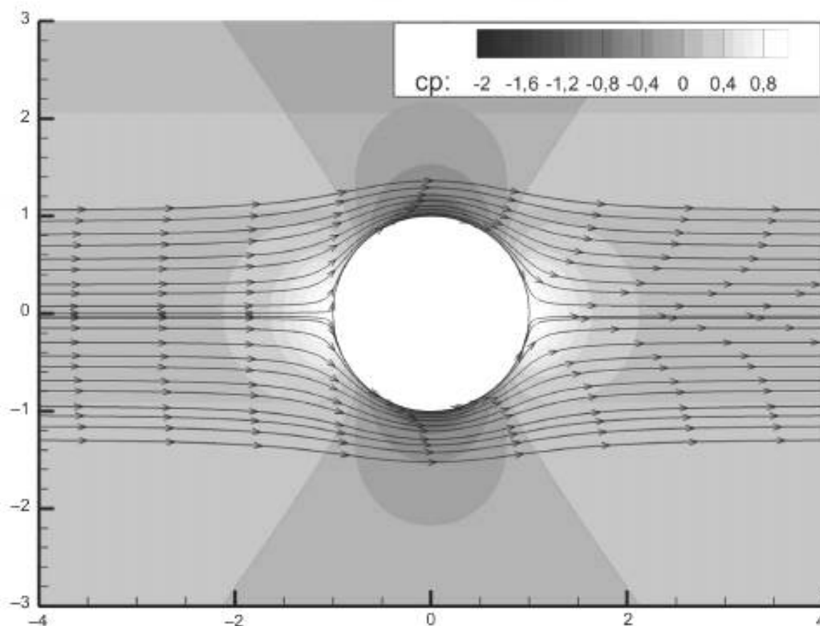
Рисунок 5 — Невязкое обтекание сферы. Осесимметричное решение при предположении о потенциальном характере обтекания
