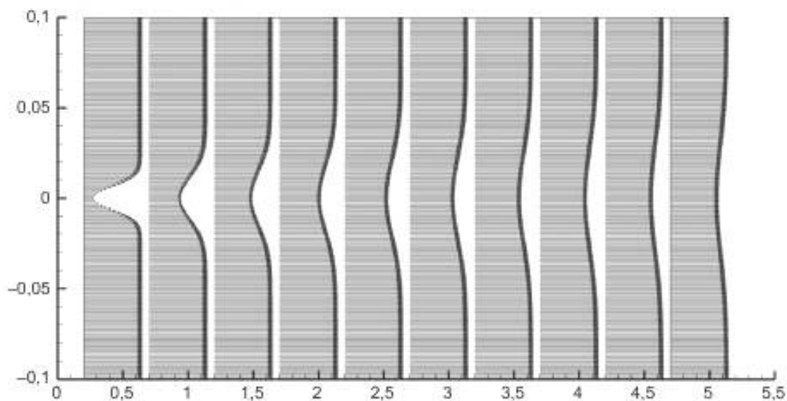
Рисунок 4 — Пример профилей скорости
