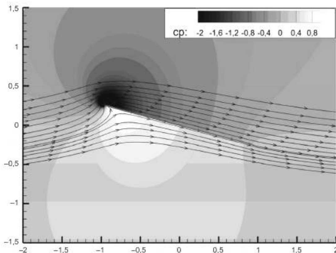
Рисунок 2 — Двумерное обтекание пластины
