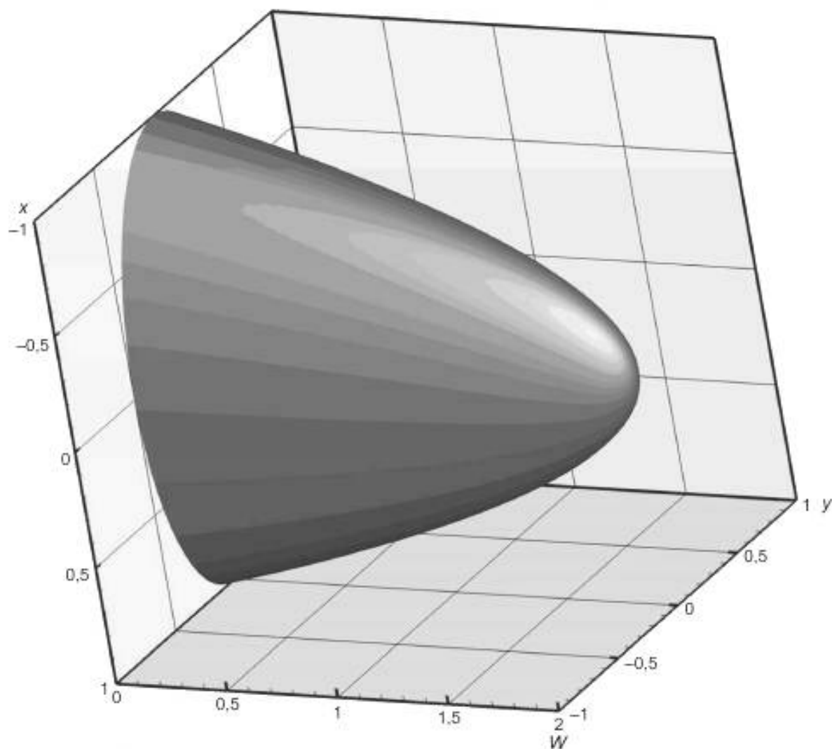
Рисунок 10 — Течение в канале с эллиптическим сечением. Решение
