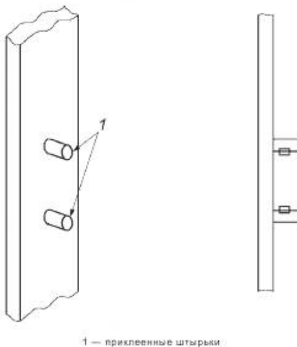
Рисунок А.1 — Пример образца для оптической тензометрии
