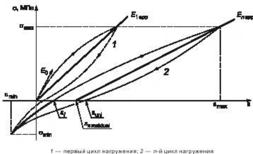
Рисунок 3 — Знакопеременный цикл нагружения
