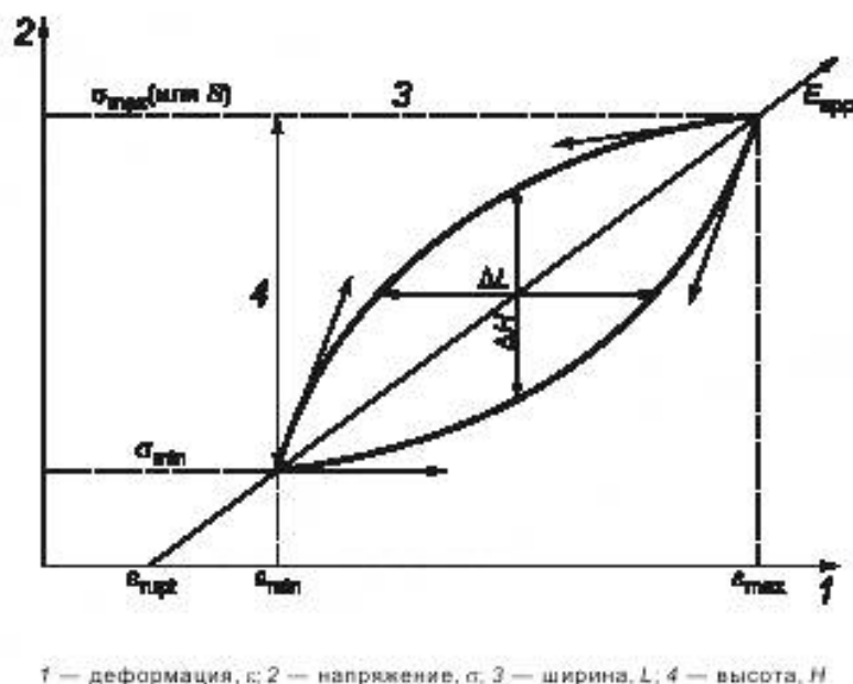
Рисунок 2 — Параметры для оценки усталостной долговечности
