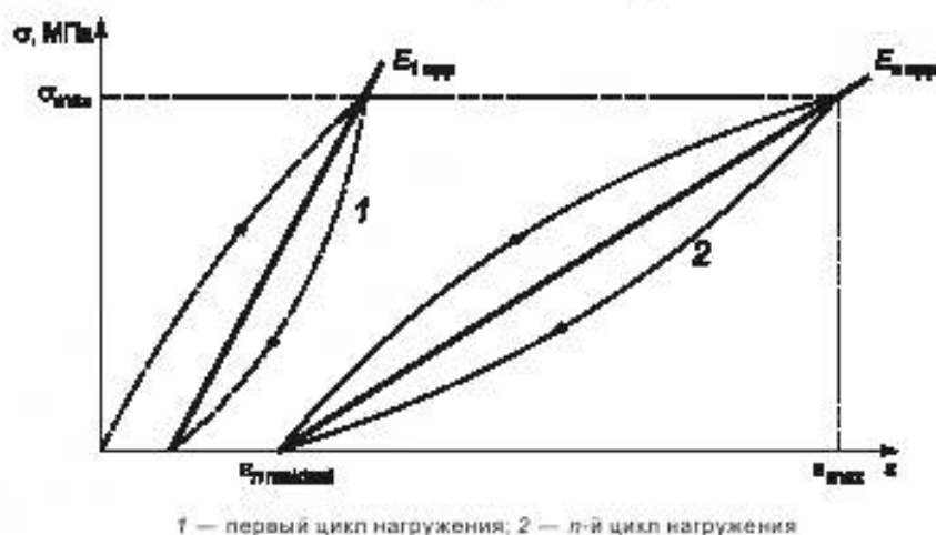
Рисунок 2 — Отнулевой цикл нагружения
