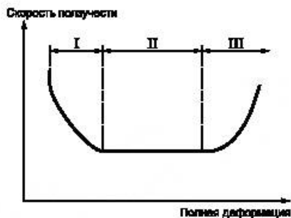
Рисунок X3.1 — Скорость ползучести
