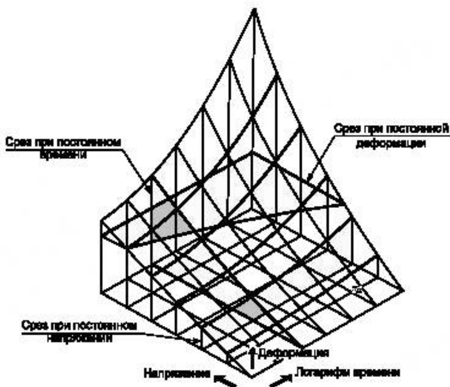
Рисунок Х4.1 — Постоянные координаты «напряжения—деформации—времени»
