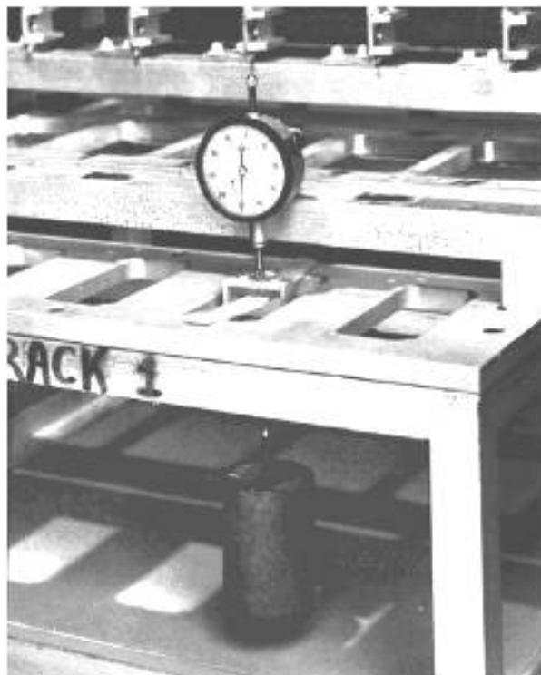
Рисунок А.1 — Испытательный стенд
