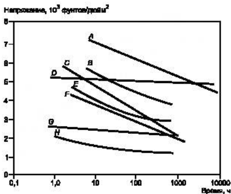
Рисунок X3.4 — Контур разрушения при ползучести
