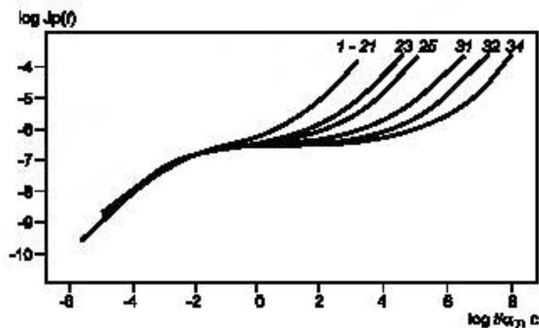
Рисунок X5.3 — Кривая податливости
