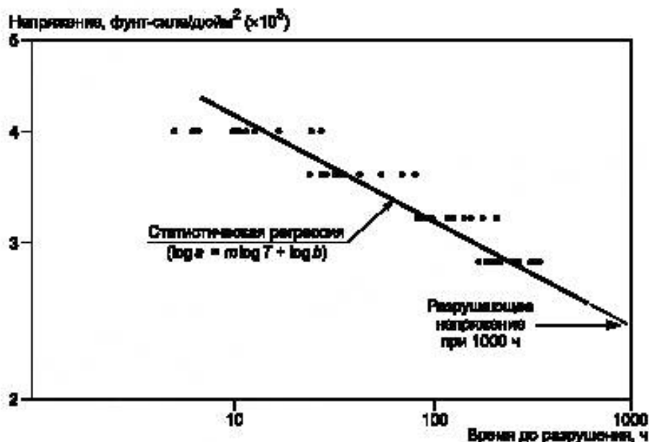
Рисунок 5 — Кривая логарифмической зависимости времени разрушения (механического разрушения)
