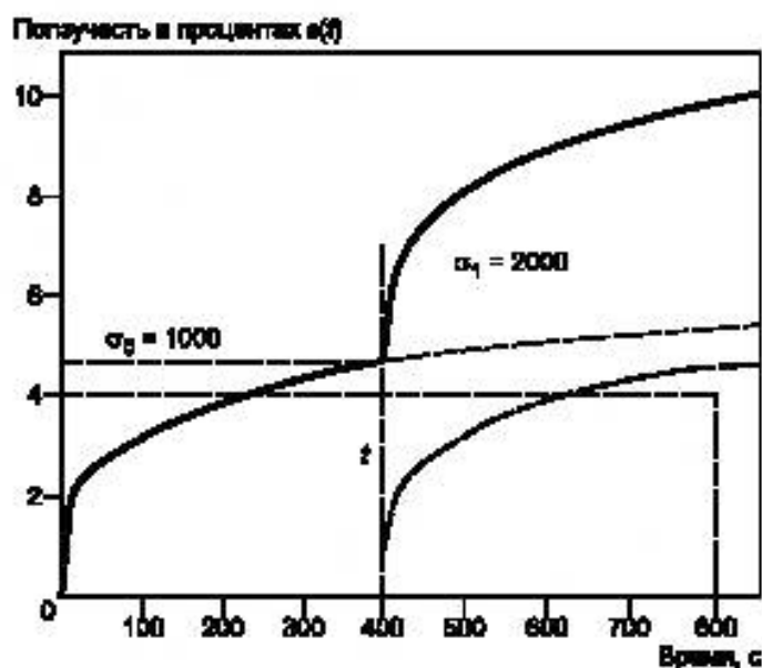
Рисунок X5.1 — Принцип Больцмана
