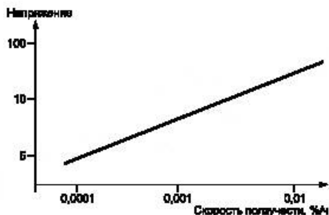
Рисунок X3.2 — Прочность при ползучести
