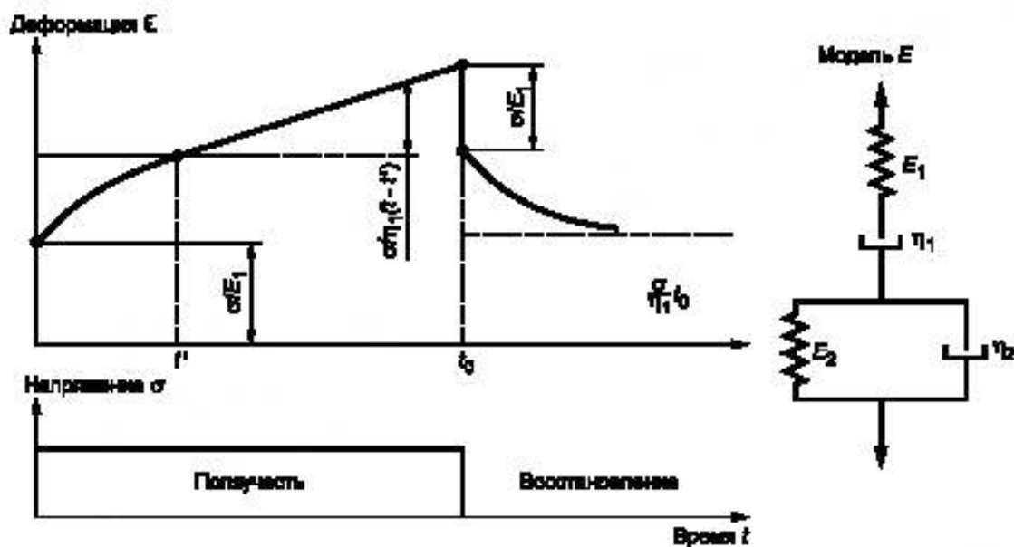
Рисунок Х6.3 — Четырехэлементная модель
