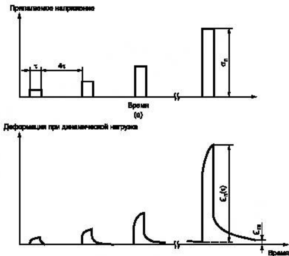
Рисунок X4.2 — Изохронные данные
