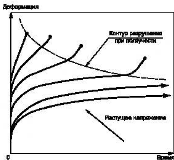
Рисунок X3.4 — Контур разрушения при ползучести
