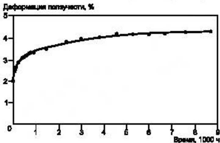
Рисунок X2.2 — Кривая ползучести при растяжении политетрафторэтилена при 650 фунтов/дюйм 2 , 23 °С. Зависимость модуля ползучести от времени
