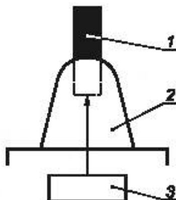
1 — образец; 2 — приспособление для испытания; 3 — датчик деформации
