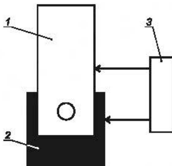
1 — приспособление для испытания; 2 — образец; 3 — датчик деформации
