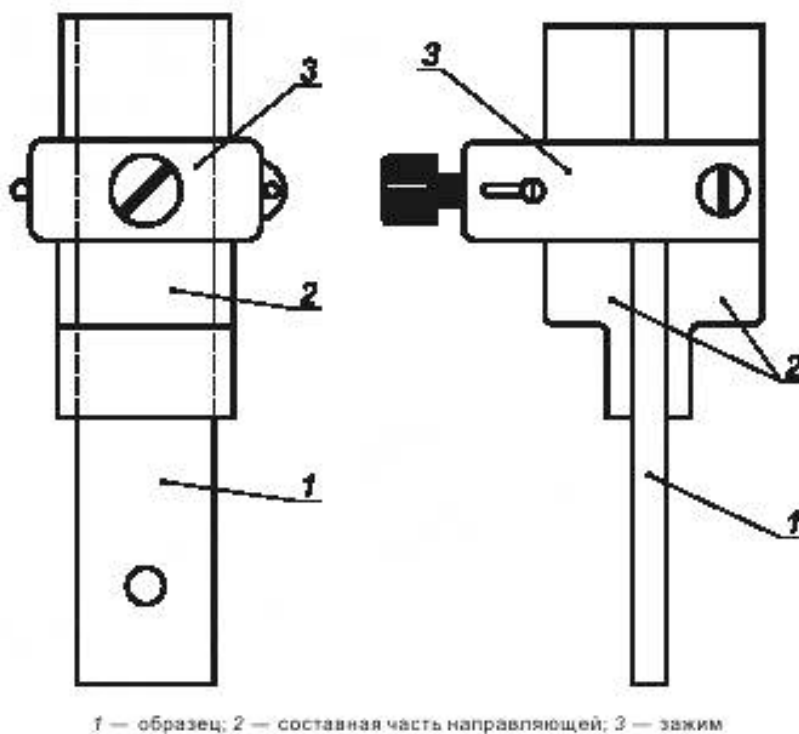
Рисунок 3 — Общий вид направляющей
