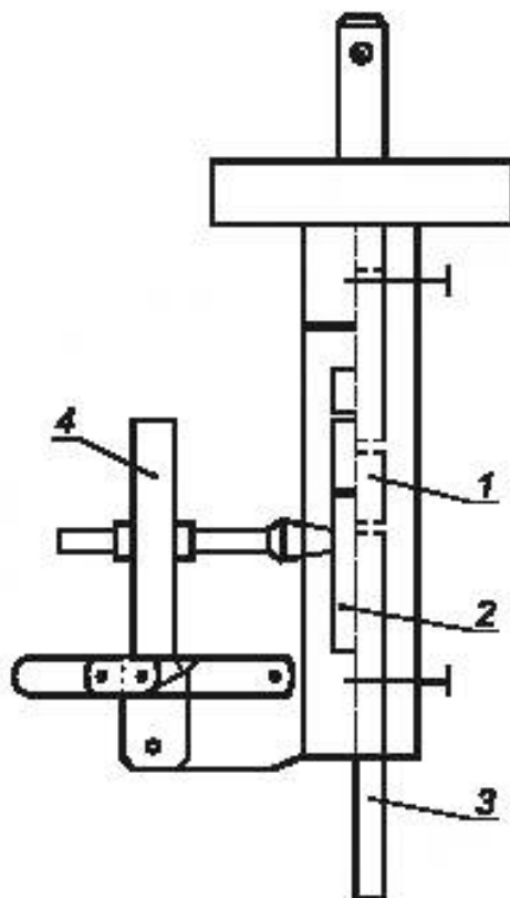
1 — образец; 2 — адаптер; 3 — нагружающее приспособление; 4 — фиксатор
