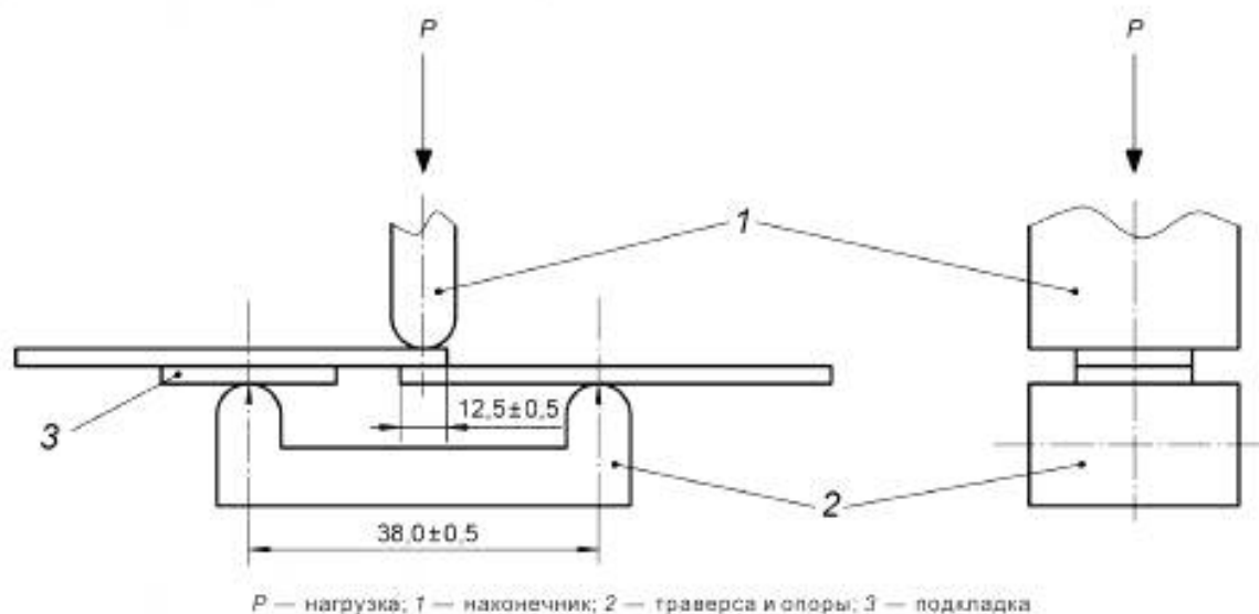
Рисунок 2 — Схема проведения испытаний
