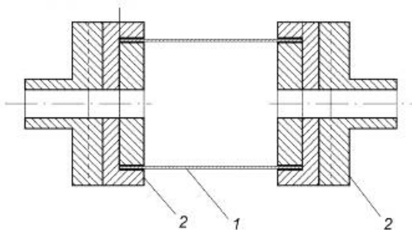
1 — образец; 2 — приспособление
