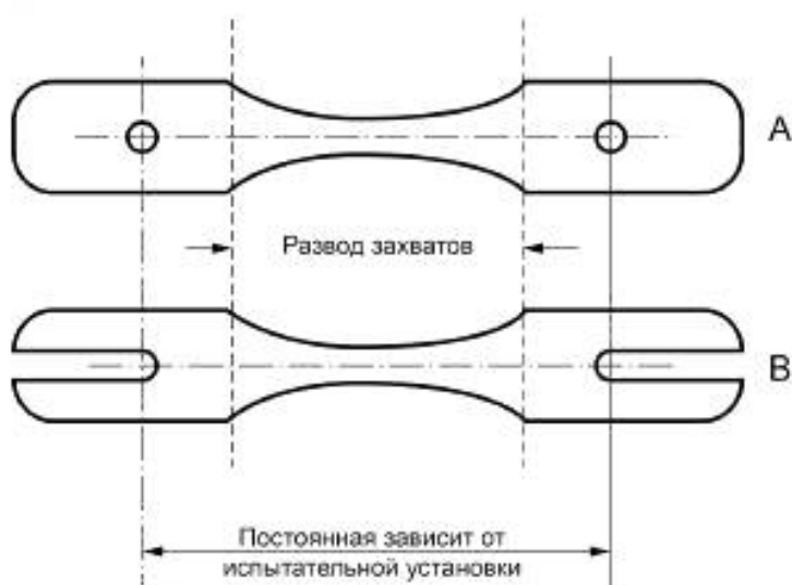
Рисунок 4 — Расположение отверстий под болты
