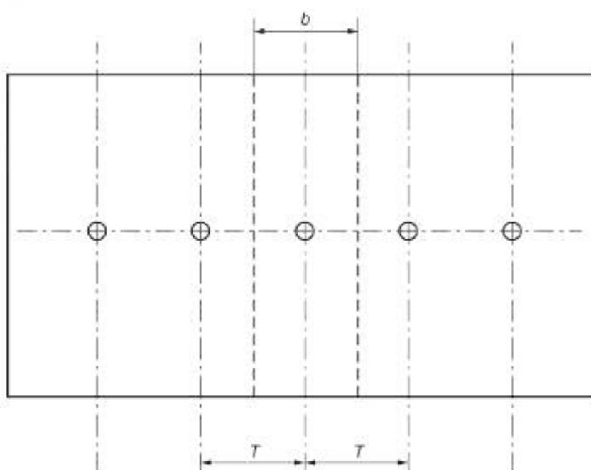
Рисунок 3 — Определение расстояния между отверстиями
