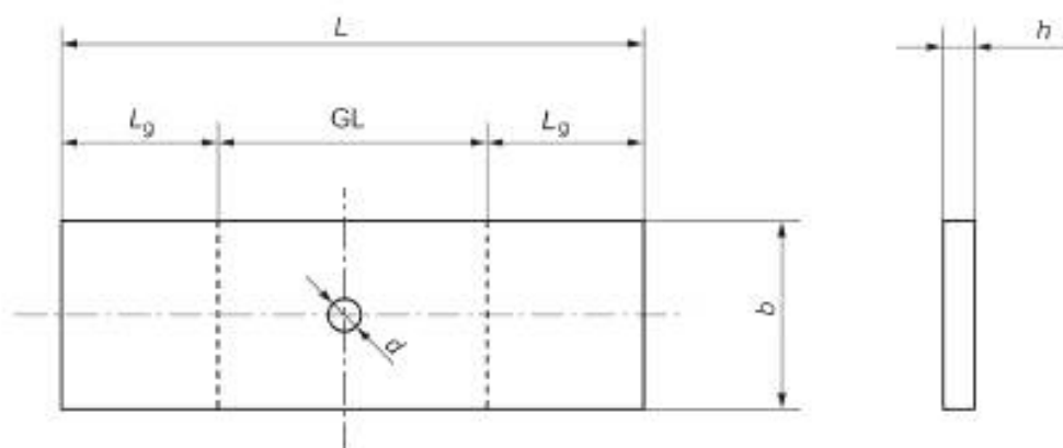
L — общая длина; GL — базовая длина; L_g — длина в захватах; h — толщина образца; b — ширина образца; d — диаметр отверстия
