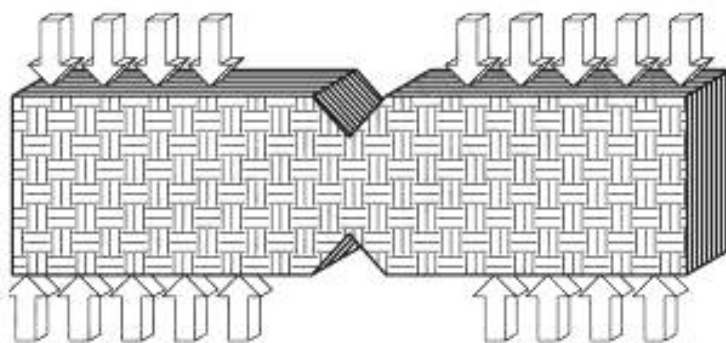
Рисунок 2 — Схема проведения испытания по методу Йосипеску
