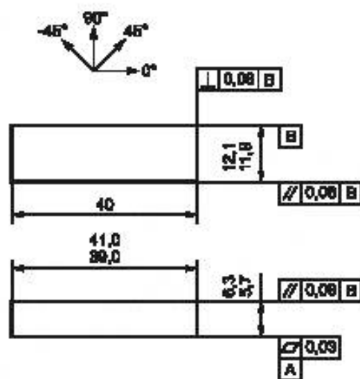
Рисунок 1 — Плоский образец
