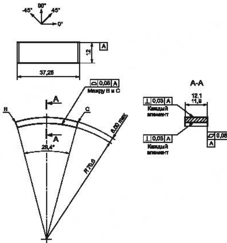
Рисунок 2 — Изогнутый образец
