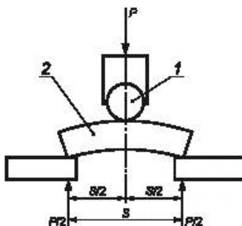
1 — наконечник; 2 — образец; P — нагрузка; S — длина пролета
