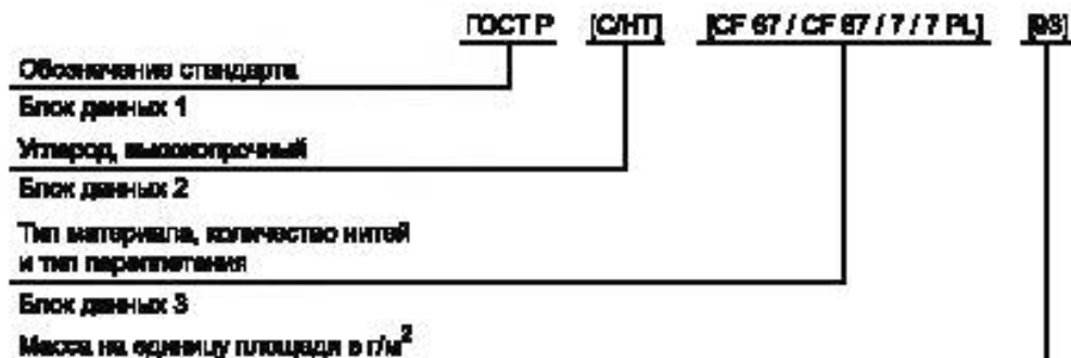
Рисунок 3 – Пример обозначения ткани из углеволокна
