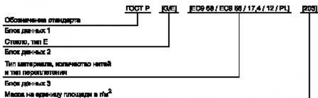
Рисунок 2 – Пример обозначения ткани из стекловолокна
