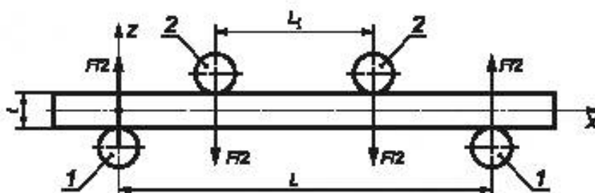
Рисунок 1 — Схема нагружения при испытании на трехточечный изгиб
