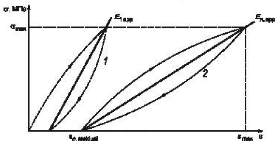
1 — первый цикл нагружения; 2 — n -й цикл нагружения
