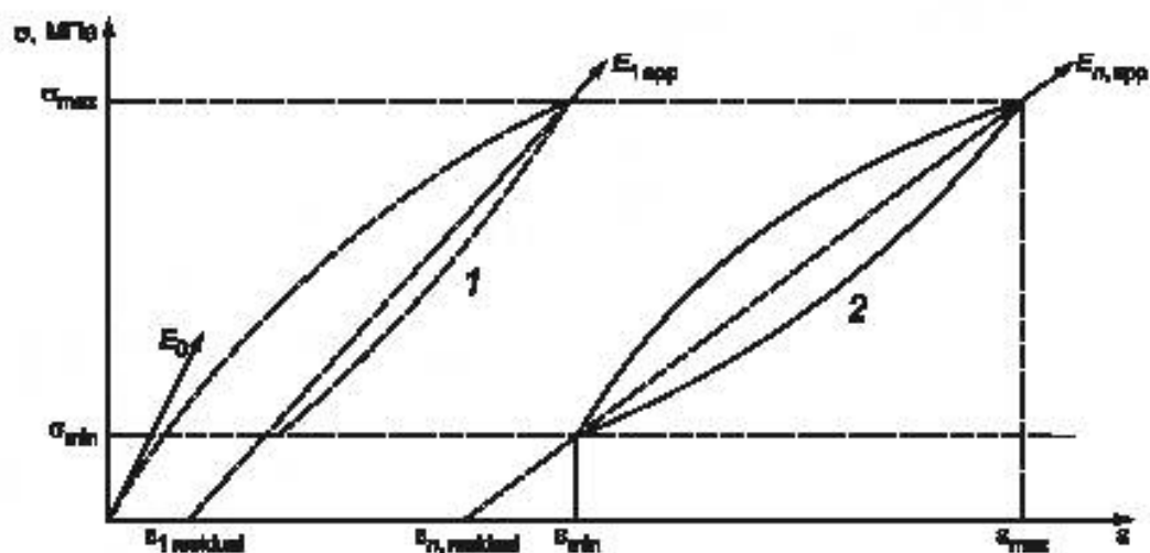
Рисунок 4 — Знакопостоянный цикл нагружения
