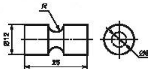
Рисунок 1 — Пример нагрузочного приспособления для испытания образцов диаметром 6 мм
