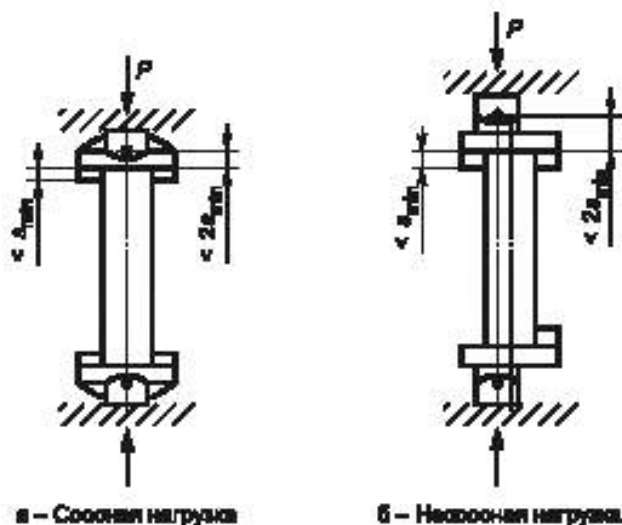
s_{\min} — наименьший размер поперечного сечения
