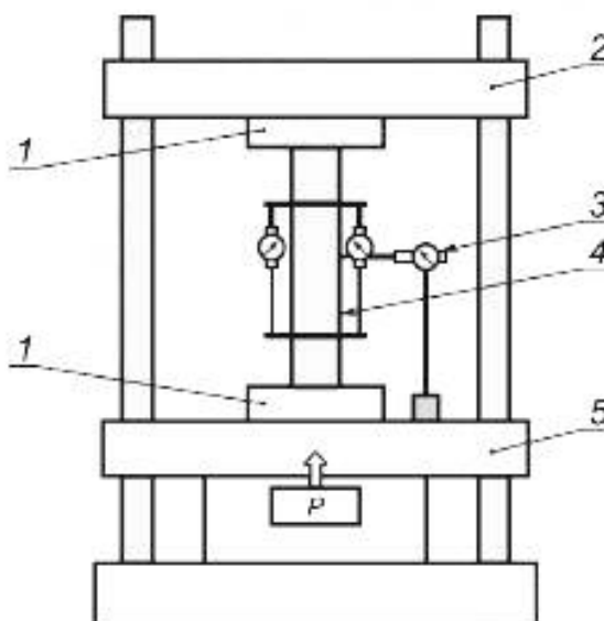
1 — нагружающая площадка; 2 — верхняя траверса; 3 — прибор для регистрации деформаций; 4 — образец; 5 — основание испытательной машины; P — нагрузка
