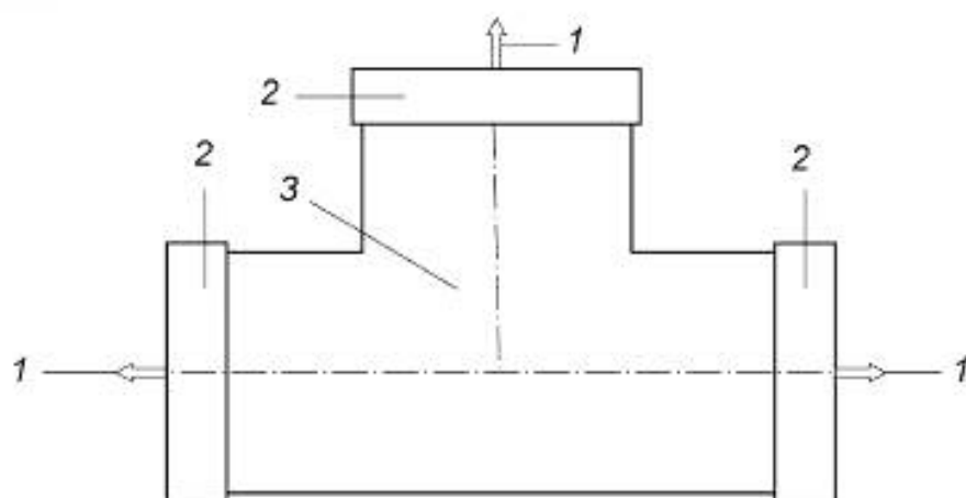
1 — осевое напряжение, воспринимаемое образцом; 2 — торцевая заглушка; 3 — фиттинг
