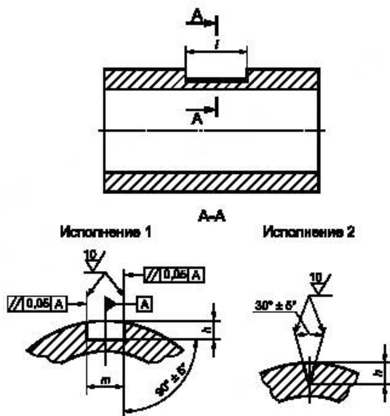
Рисунок 2 — Искусственный отражатель типа риски
