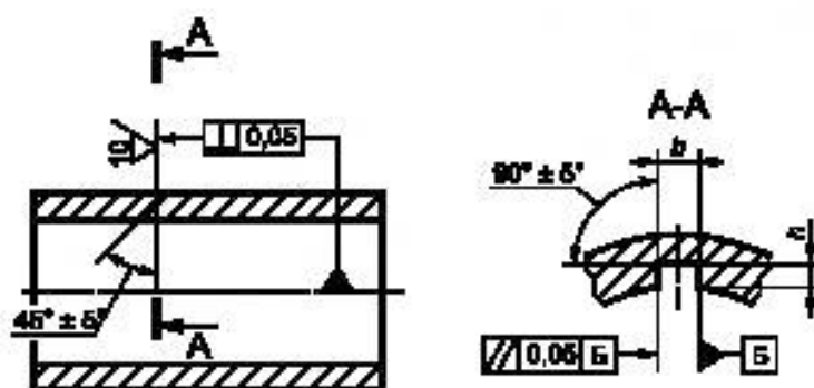
Рисунок 11 — Искусственный отражатель типа зарубки
