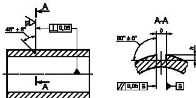
Рисунок 12 — Искусственный отражатель типа зарубки
