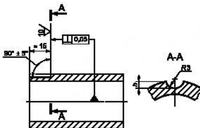
Рисунок 10 — Искусственный отражатель типа сегментного отражателя
