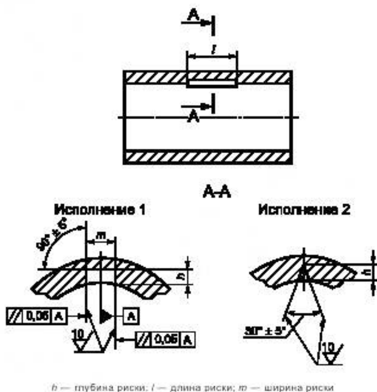
Рисунок 1 — Искусственный отражатель типа риски
