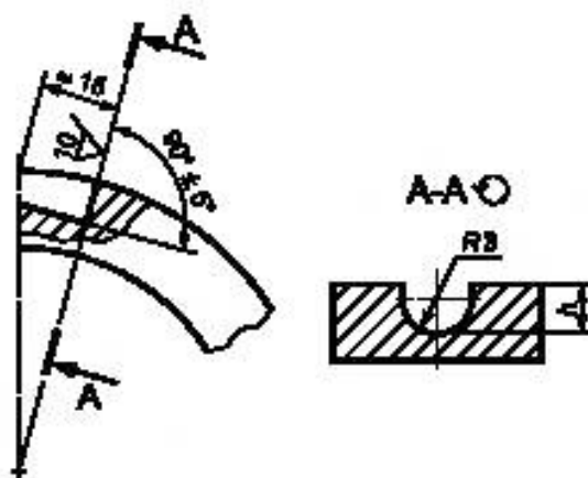
Рисунок 4 — Искусственный отражатель типа сегментного отражателя
