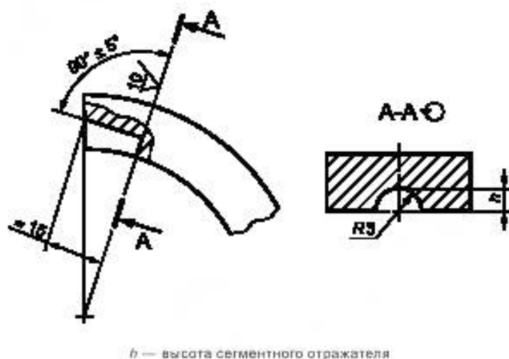
Рисунок 3 — Искусственный отражатель типа сегментного отражателя
