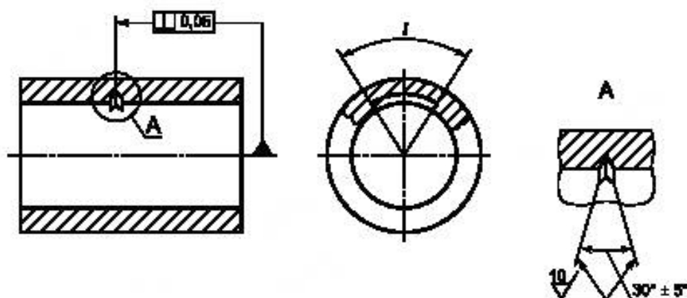
Рисунок 7 — Искусственный отражатель типа риски
