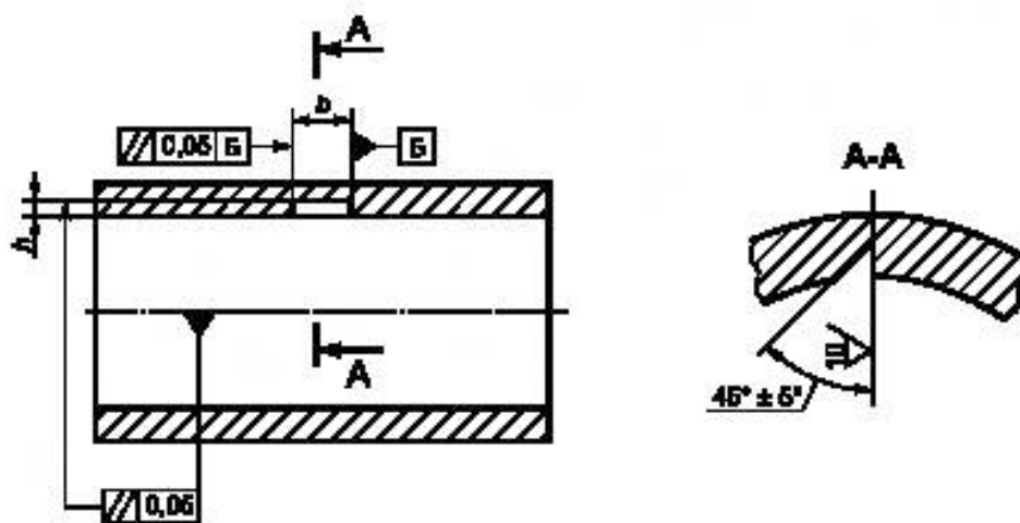
Рисунок 5 — Искусственный отражатель типа зарубки
