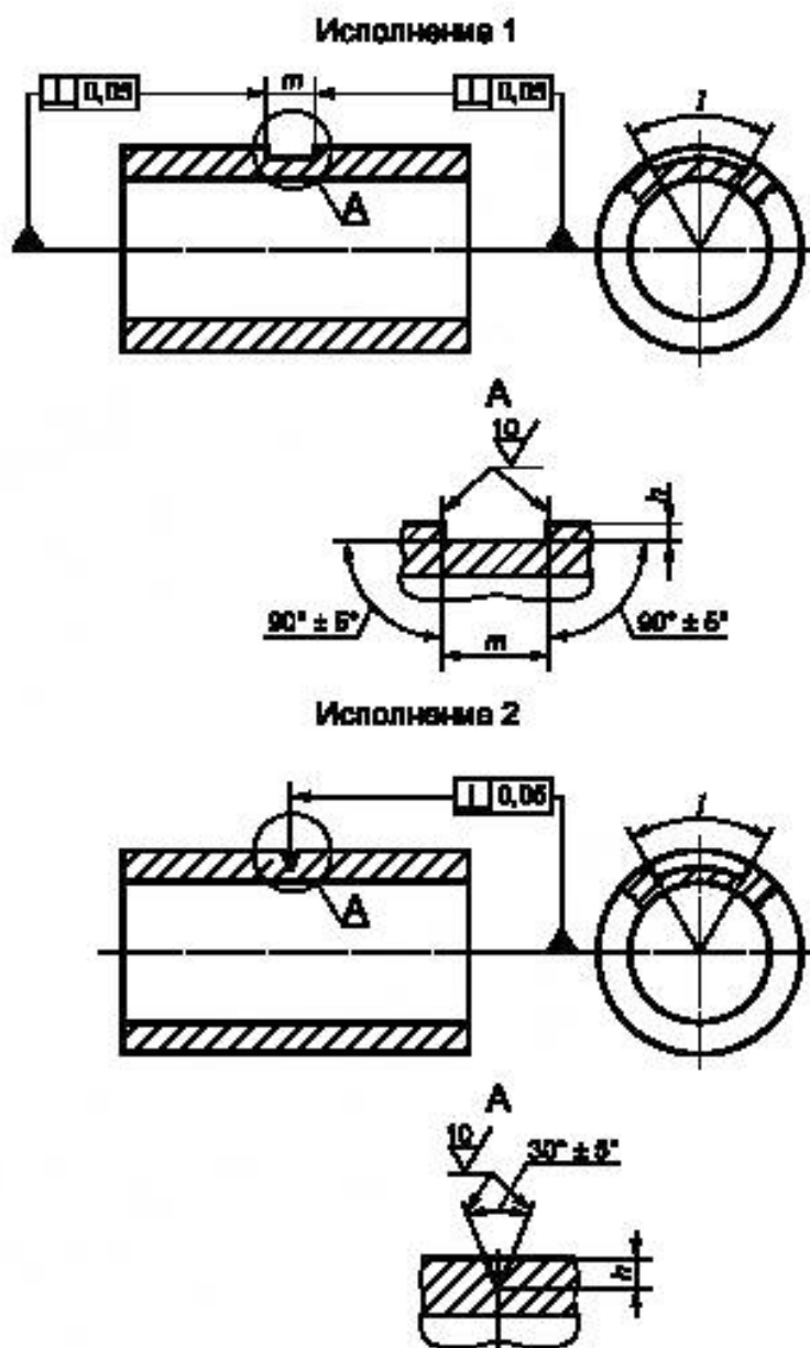
Рисунок 8 — Искусственный отражатель типа риски
