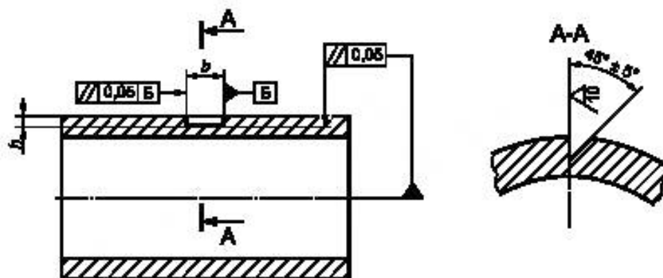
Рисунок 6 — Искусственный отражатель типа зарубки
