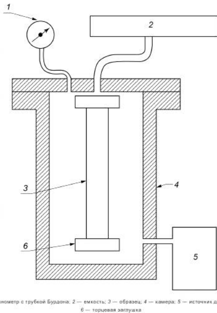
Рисунок 1 — Схема испытания, обеспечивающего воздействие на образец внешнего давления в кольцевом и продольном направлении
