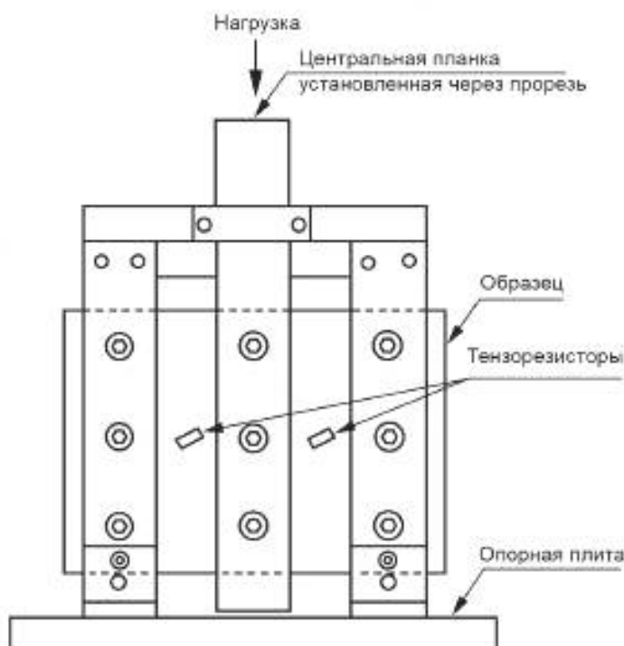
Рисунок 3 — Метод В. Эскиз приспособления
