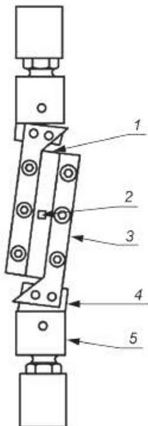
1 — образец; 2 — тензорезистор; 3 — зажимные планки; 4 — выравнивающая плитка; 5 — скоба
