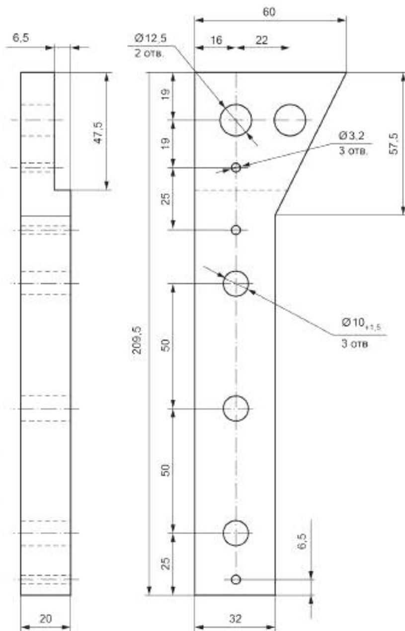
Рисунок ДА.1 — Эскиз зажимных планок
