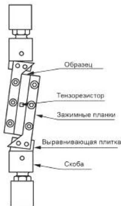
Рисунок 1 — Метод А. Приспособление для сдвига
