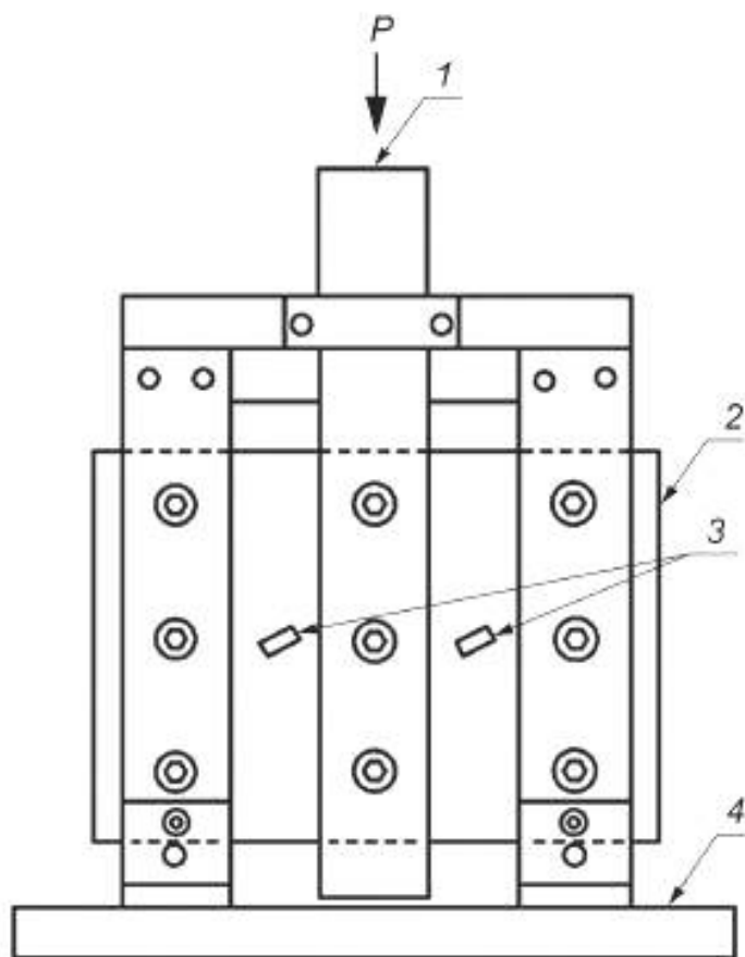
P — нагрузка, 1 — центральная планка, установленная через прорезь; 2 — образец; 3 — тензорезисторы; 4 — опорная плита
