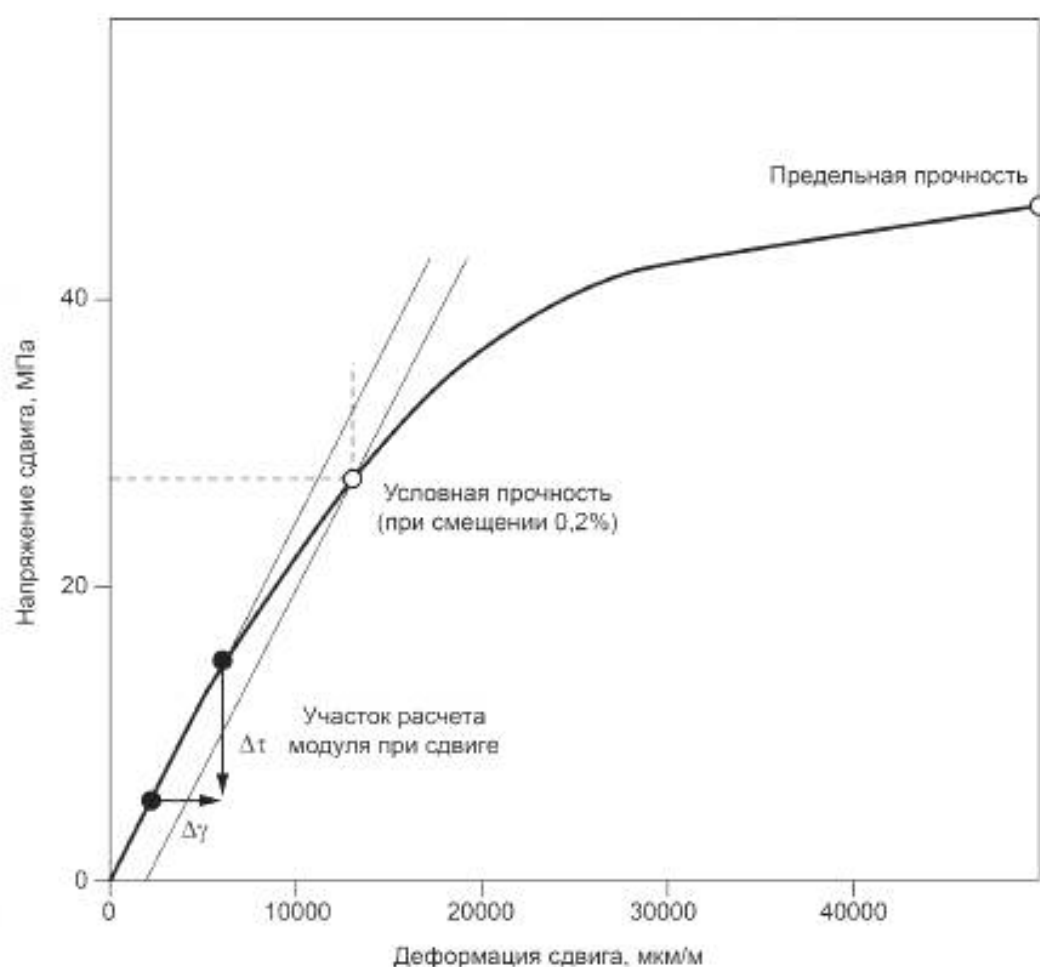
Рисунок 7 — Пример кривой «напряжение сдвига — деформация сдвига»
