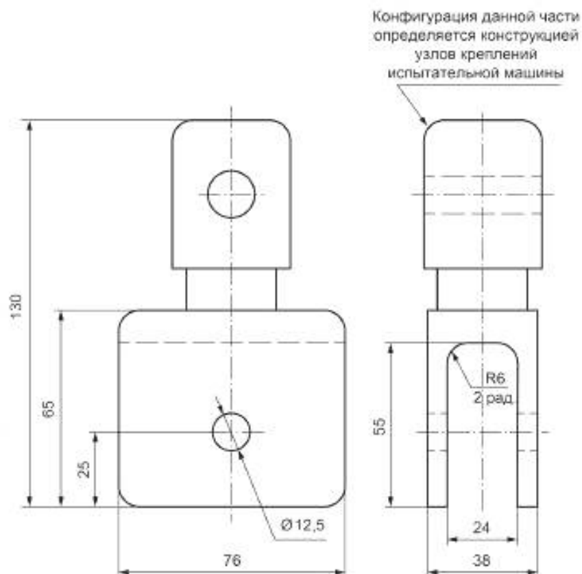
Рисунок ДА.2 — Эскиз скобы
