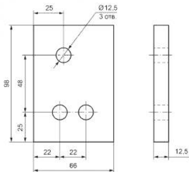
Рисунок ДА.3 — Эскиз выравнивающей пластины
