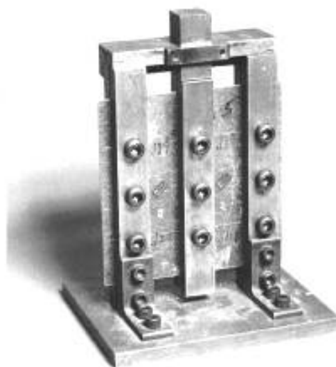
Рисунок 4 — Метод В. Фотография приспособления
