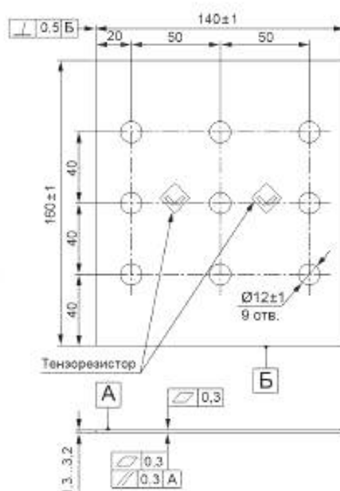
Рисунок 6 — Эскиз образца, испытываемого по методу В
