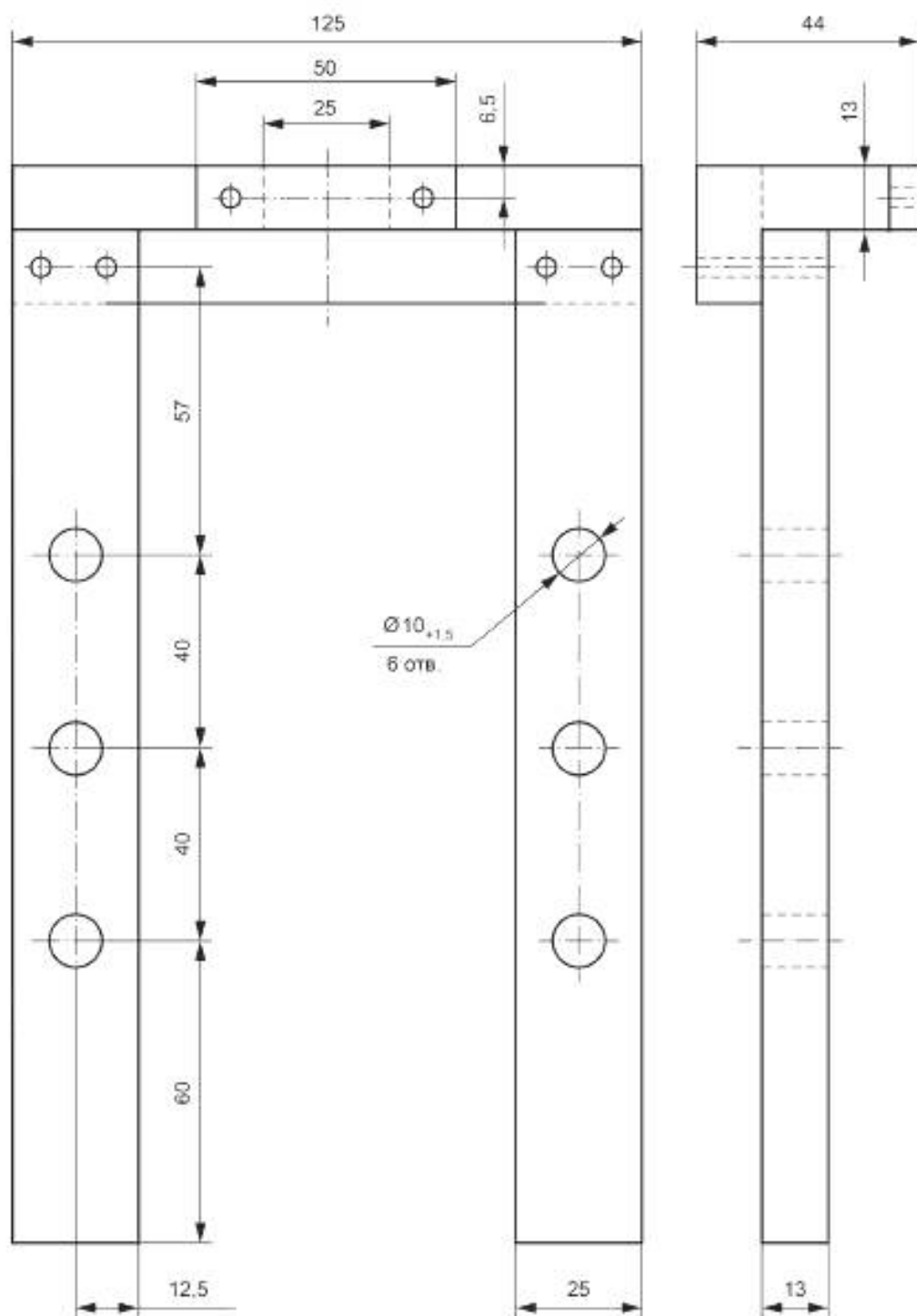
Рисунок ДБ.2 — Эскиз крайних планок с верхней перекладиной
