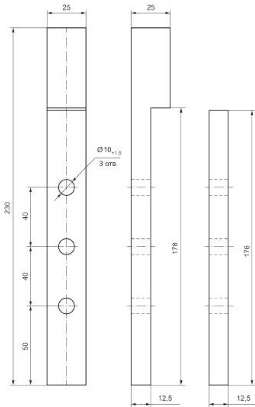
Рисунок ДБ.1 — Эскиз центральной пары планок
