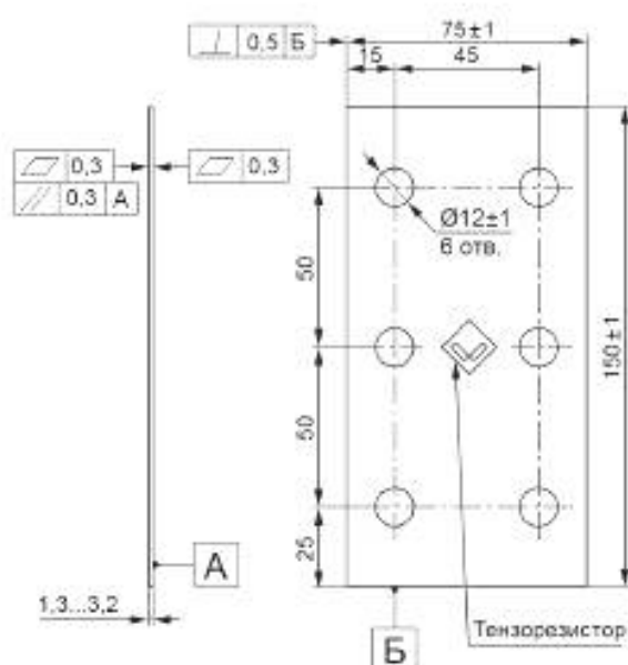
Рисунок 5 — Эскиз образца, испытываемого по методу А
