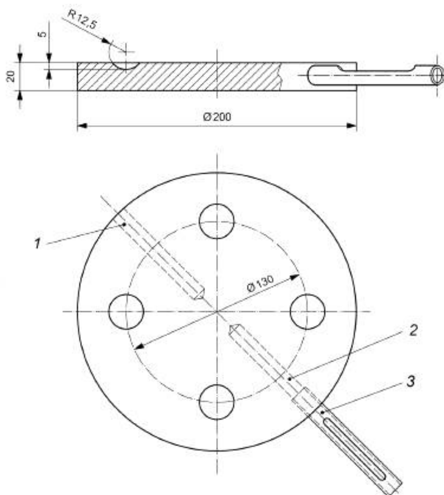
1 — отверстие для термодары устройства контроля температуры; 2 — отверстие для термометра; 3 — защитная металлическая трубка для термометра
