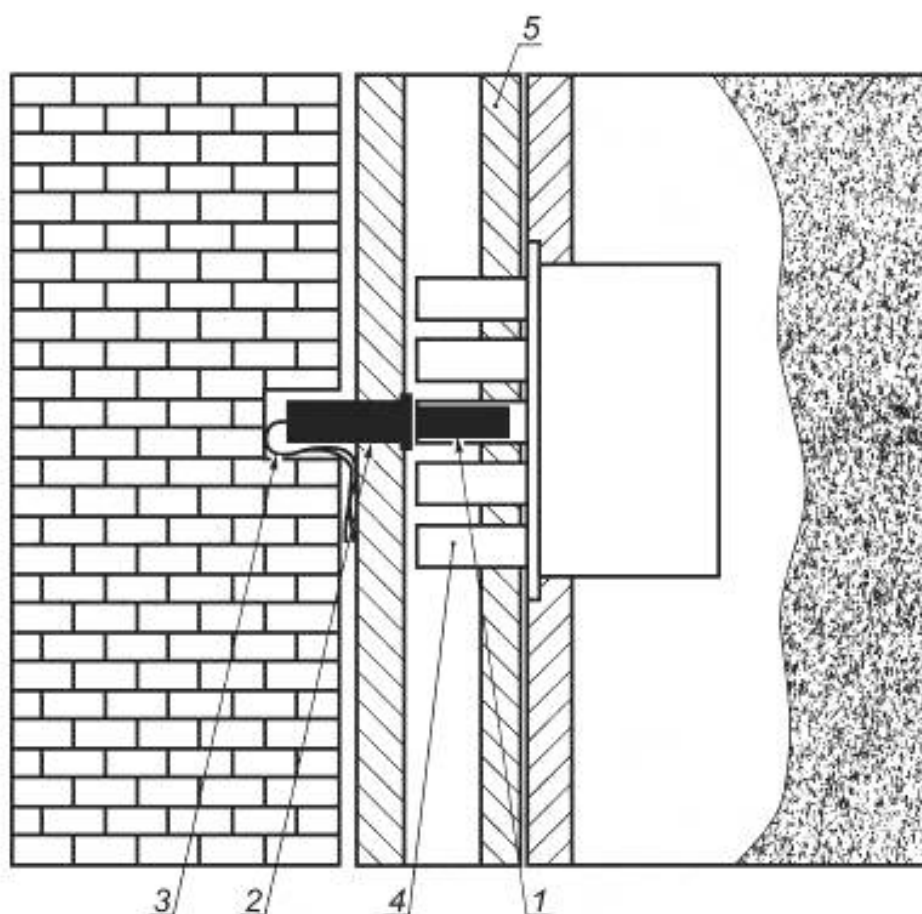
1 — магнит; 2 — геркон; 3 — провод; 4 — ригель; 5 — коробка
