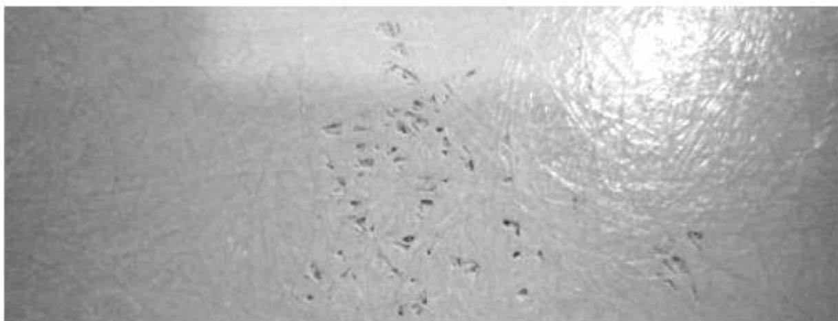
Рисунок А.27 — Пустоты в смоле
