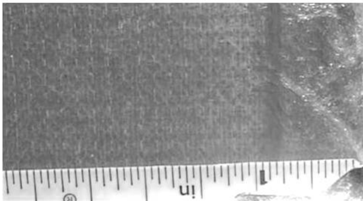
Рисунок А.13 — Проступление армирующего материала/Смещение вуали
