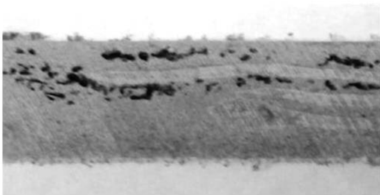
Рисунок А.23 — Внутренняя пористость
