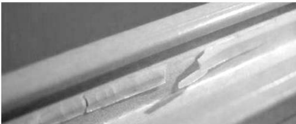
Рисунок А.33 — Отслоение
