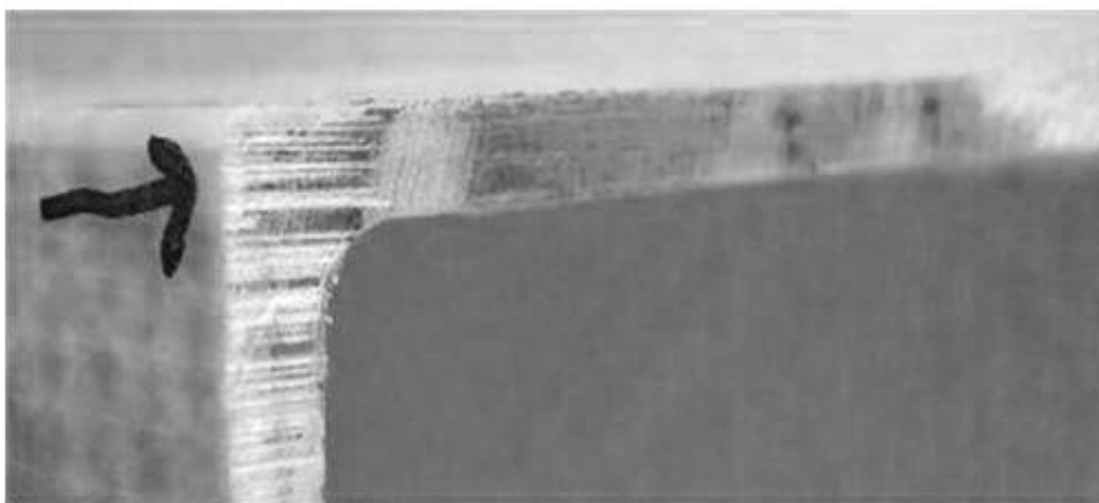
Рисунок А.29 — Пилообразное подгорание
