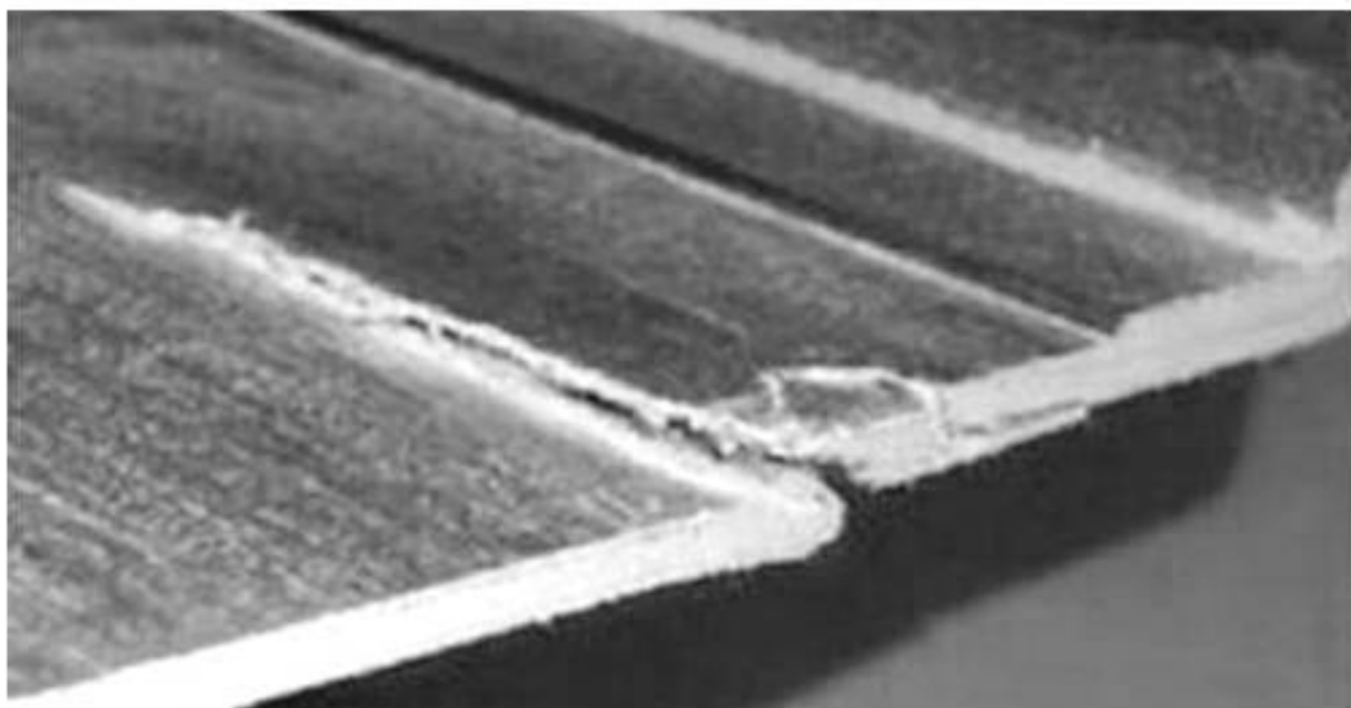
Рисунок А.17 — Разрыв
