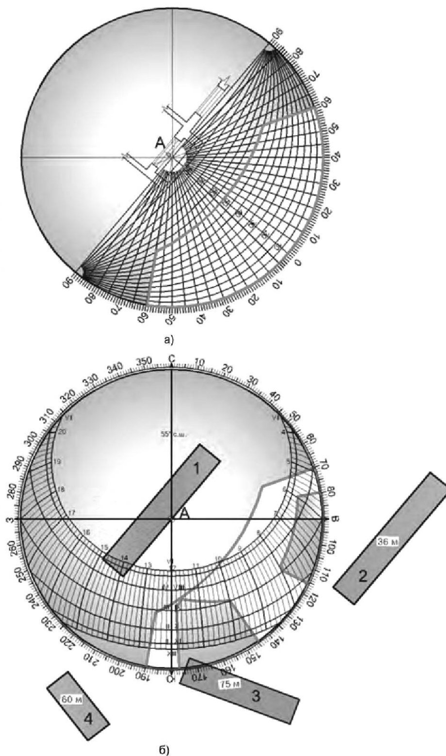
Рисунок Б.2 — Схема построения картограммы окна с лоджией (а) и схема расчета продолжительности инсоляции в помещении с лоджией в сложившейся застройке с помощью солнечной карты (б)
