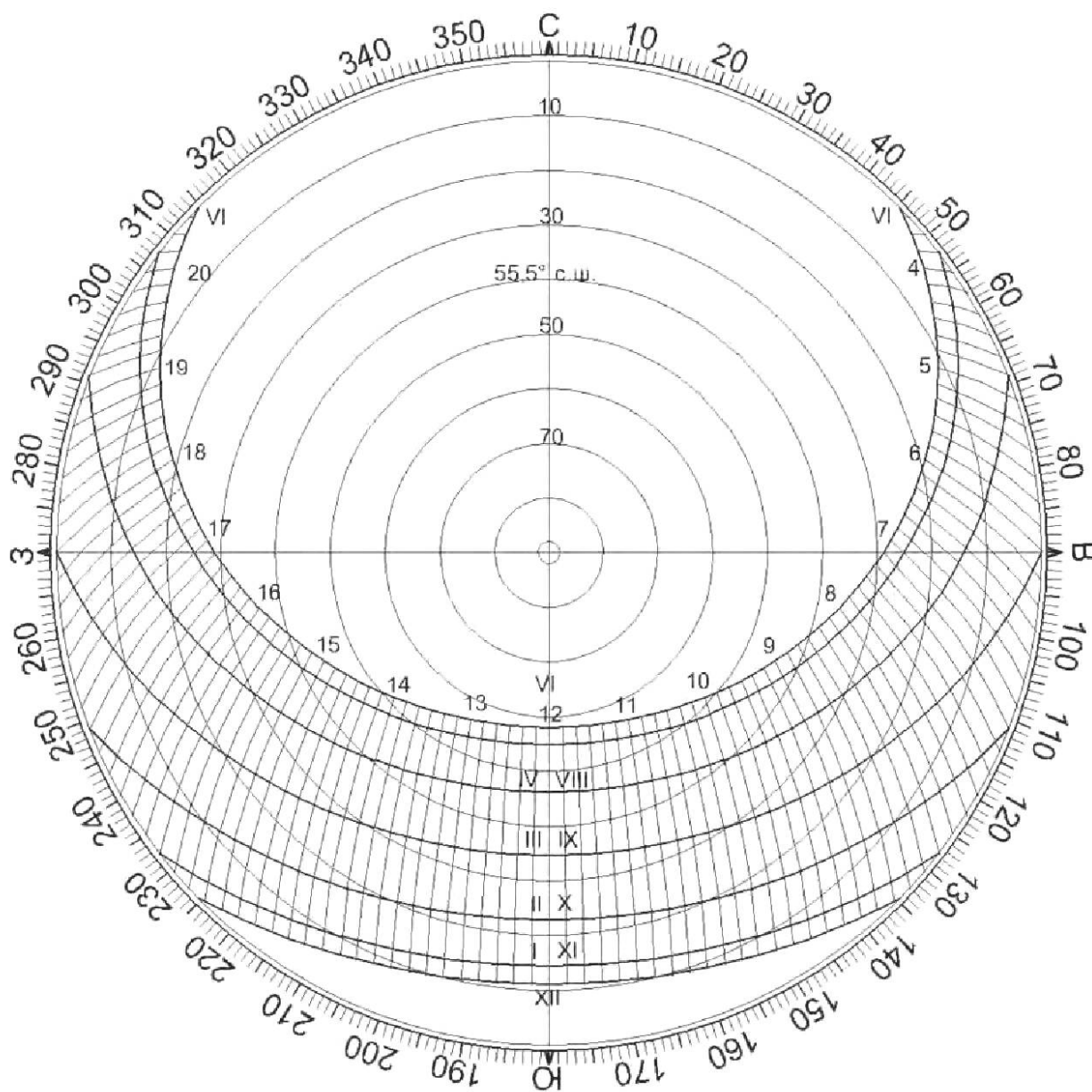
Рисунок Г.14 — Солнечная карта с равнопромежуточными альмукантаратами для города Москвы на 55,5° с. ш.
