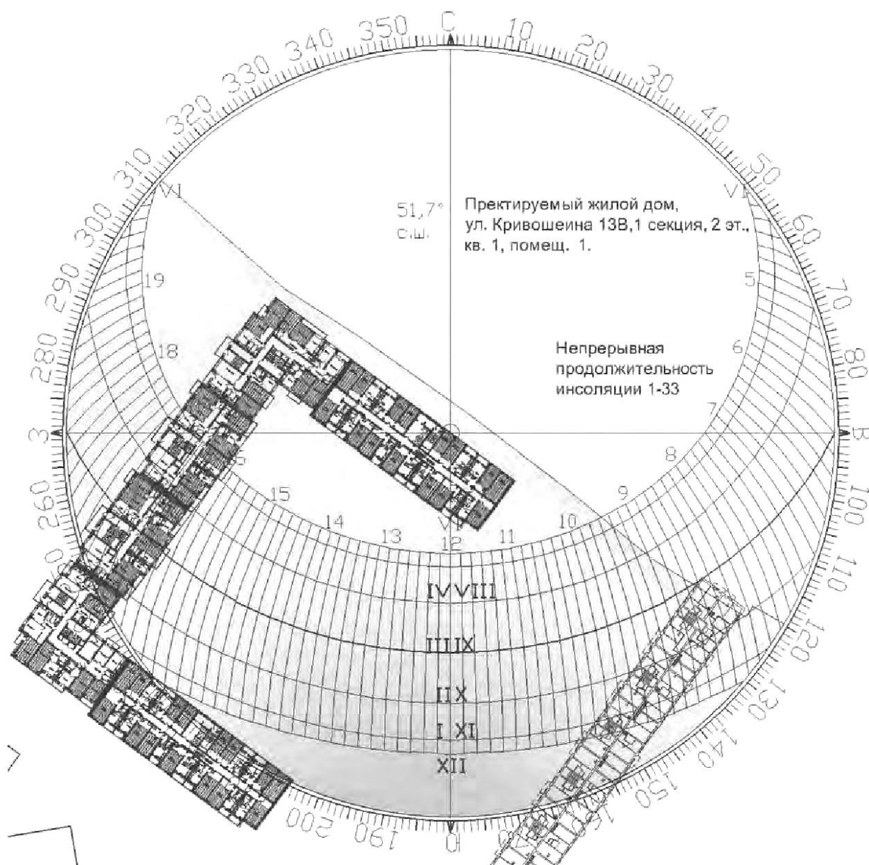
Рисунок Д.2 — Пример представления результатов графического расчета продолжительности инсоляции с помощью солнечной карты
