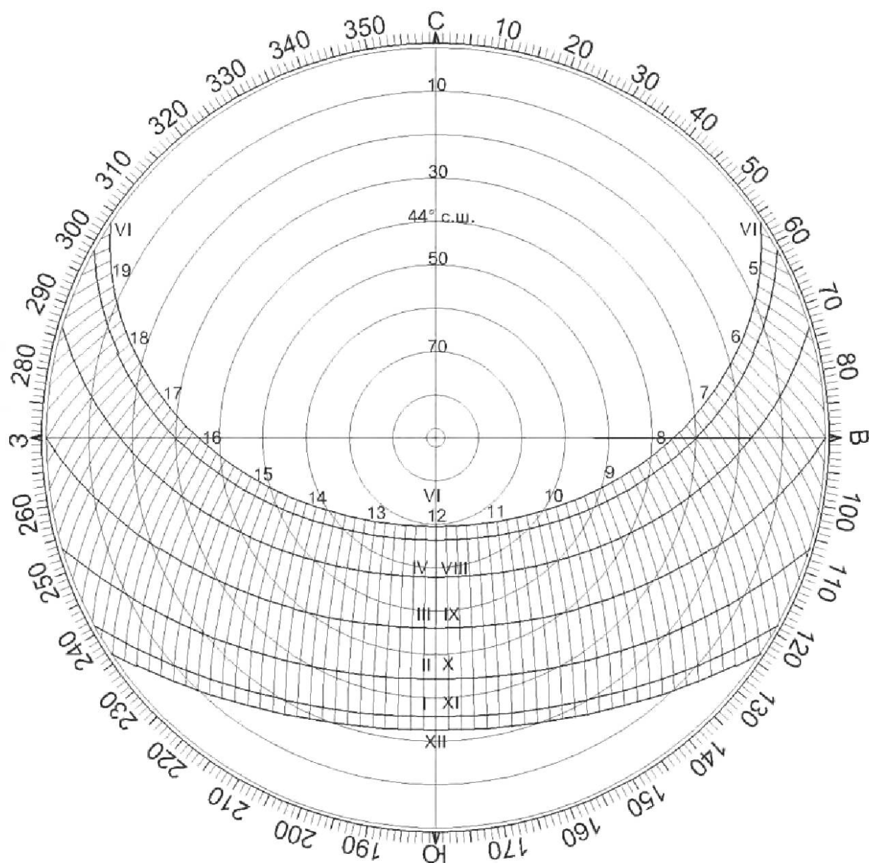
Рисунок Г.3 — Солнечная карта с равнопромежуточными альмукантаратами для территории Российской Федерации, расположенной на 44° с. ш.
