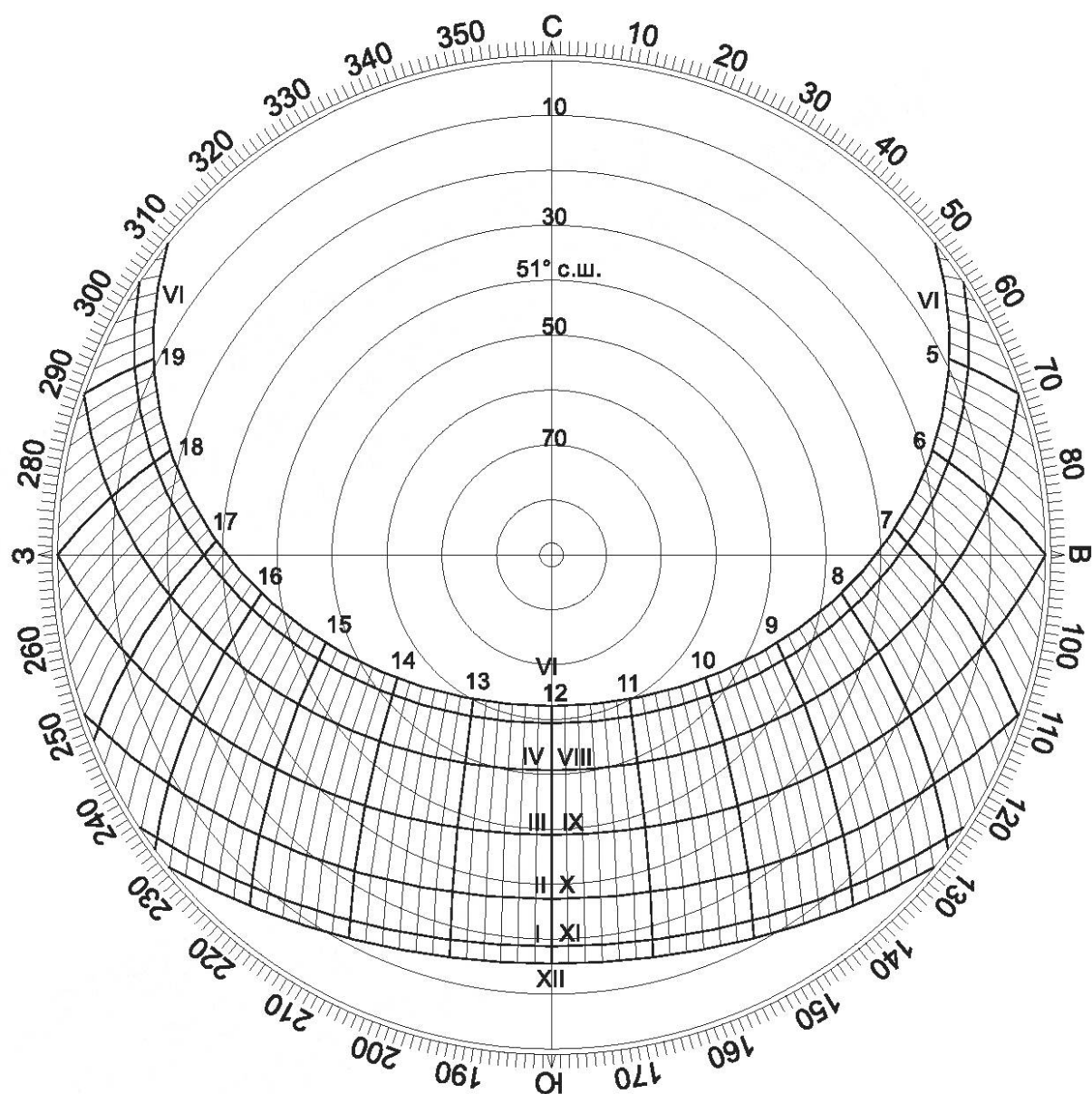
Рисунок Г.56 — Солнечная карта с равнопромежуточными альмукантаратами для территории Российской Федерации, расположенной на 51° с. ш.»;
