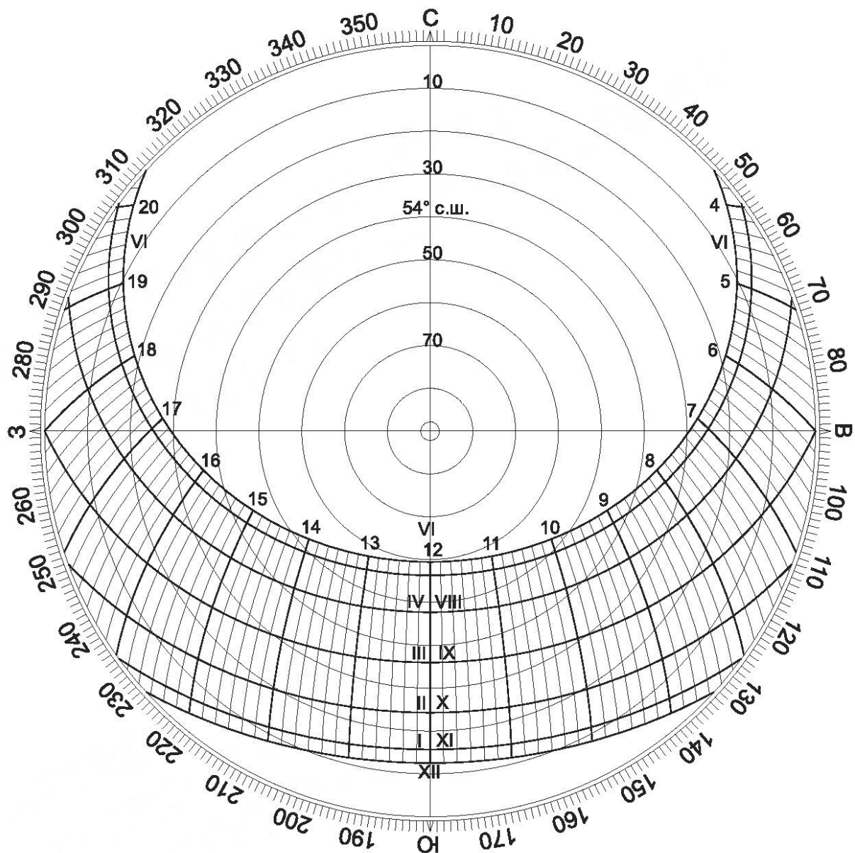
Рисунок Г.66 — Солнечная карта с равнопромежуточными альмукантаратами для территории Российской Федерации, расположенной на 54^\circ с. ш.
