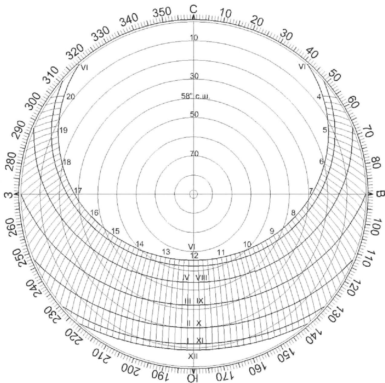
Рисунок Г.7 — Солнечная карта с равнопромежуточными альмукантаратами для территории Российской Федерации, расположенной на 58° с. ш.
