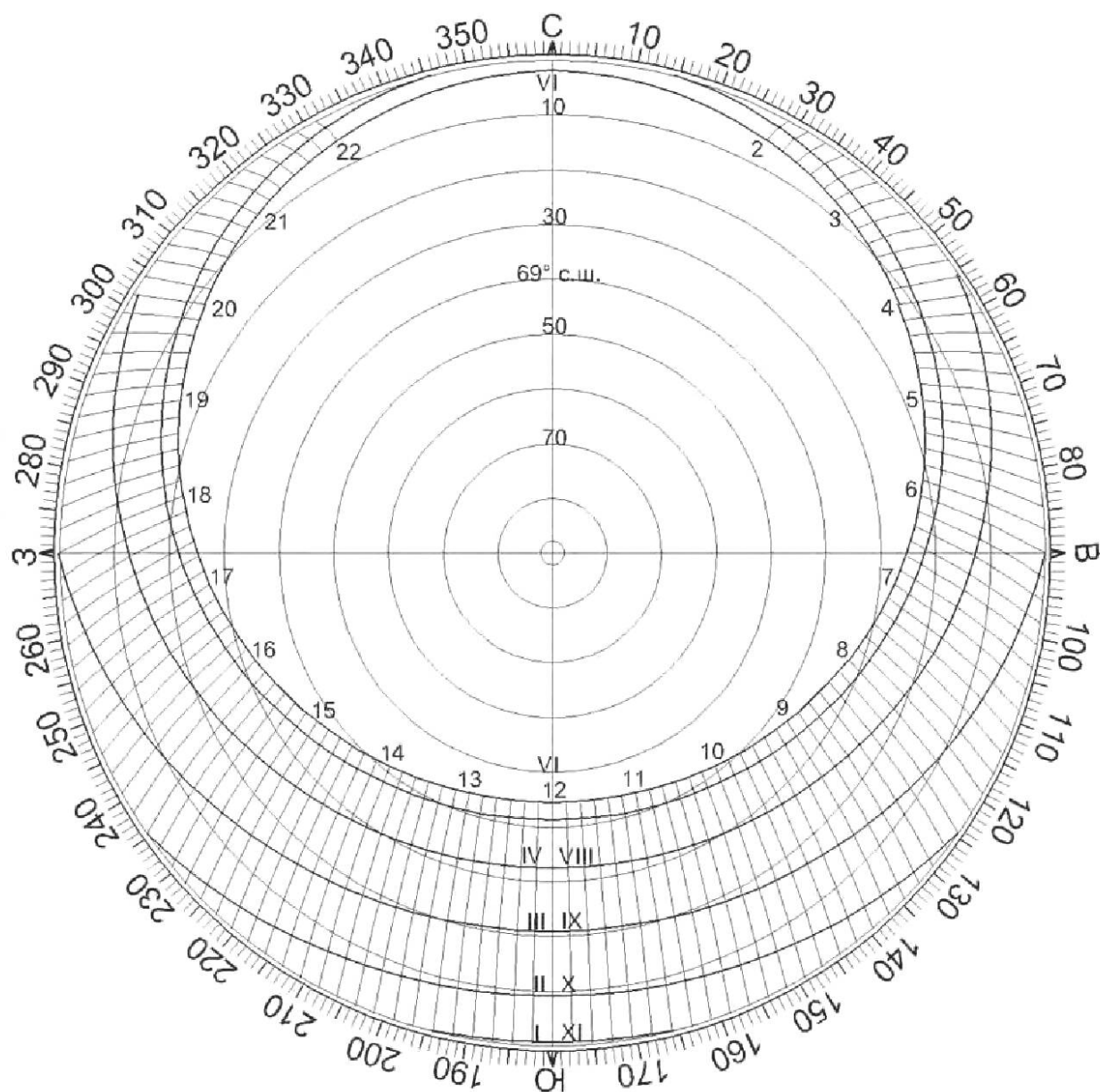
Рисунок Г.11 — Солнечная карта с равнопромежуточными альмукантаратами для территории Российской Федерации, расположенной на 69° с. ш.
