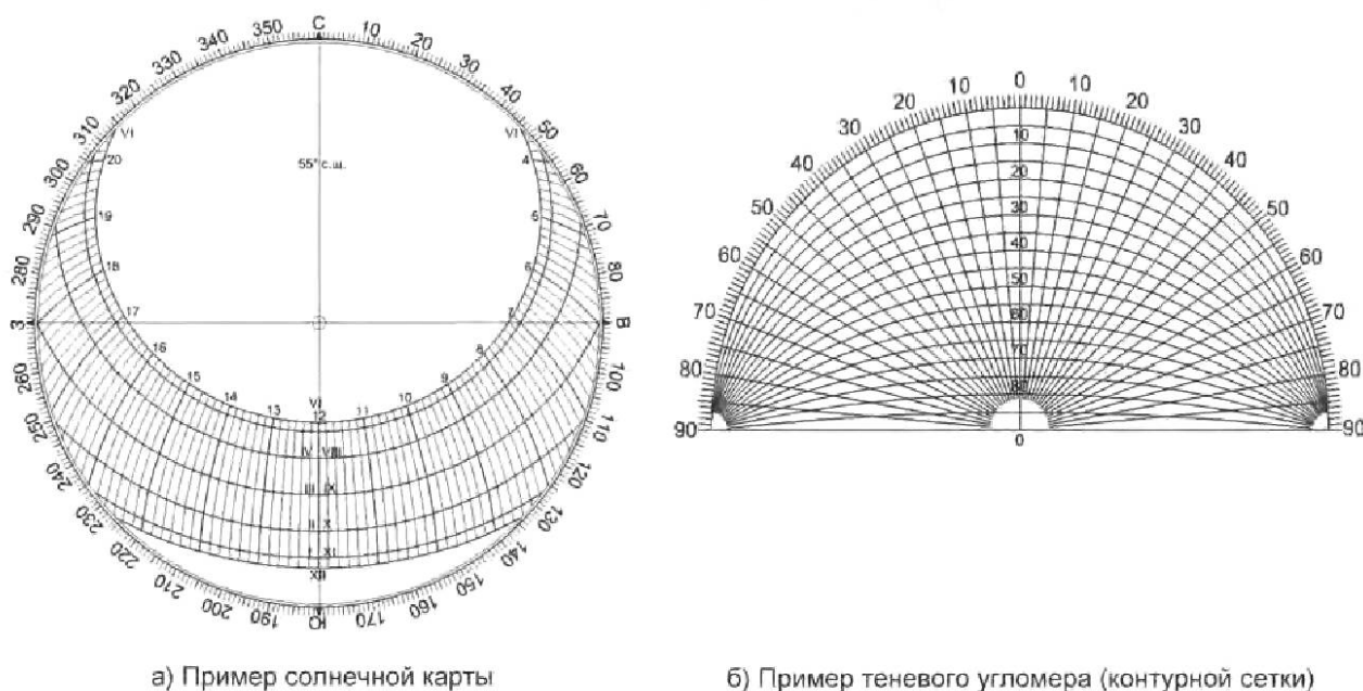
Рисунок 2 — Солнечная карта, разработанная применительно ко всем месяцам года, и теневой угломер
