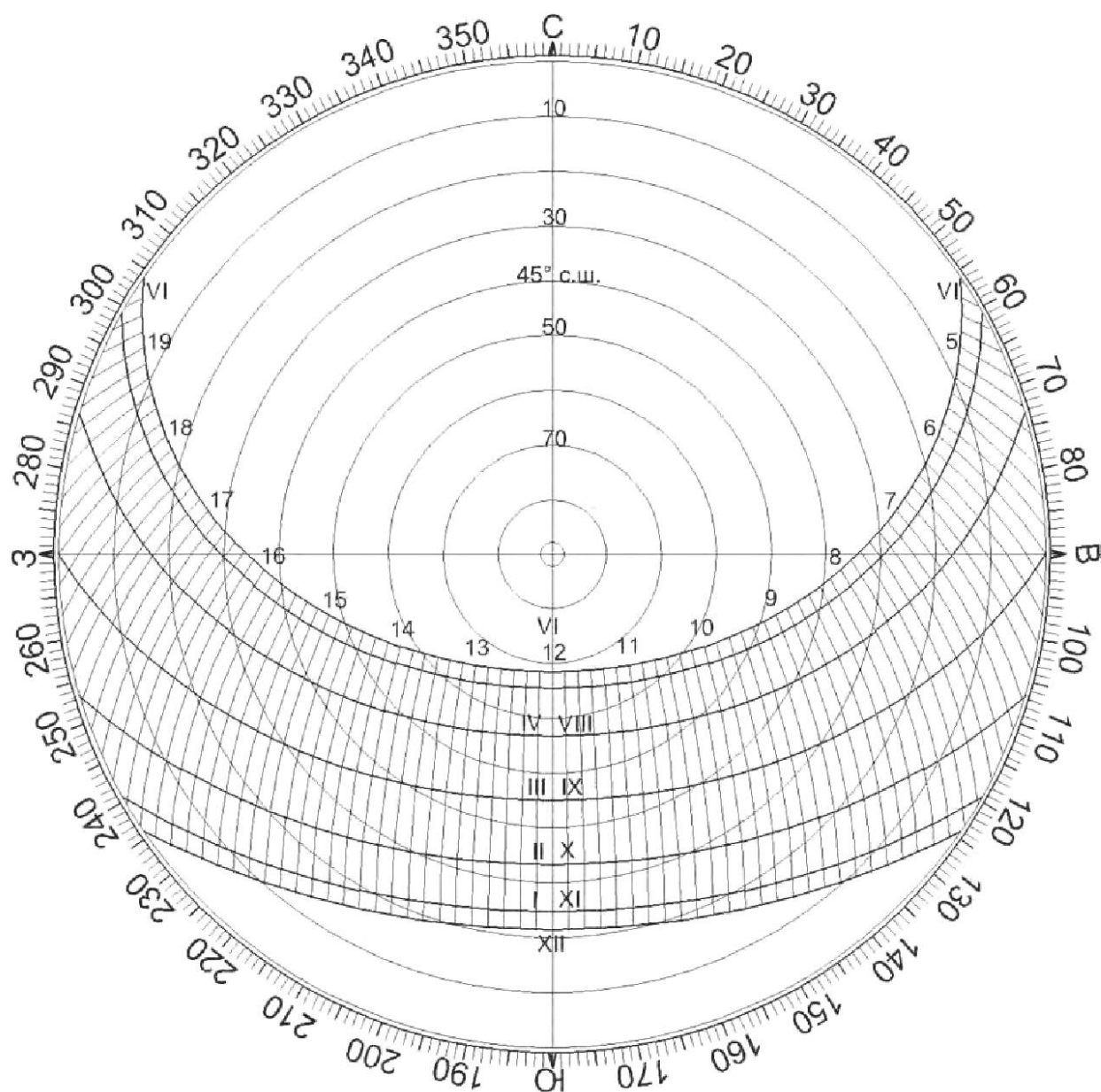
Рисунок Г.4 — Солнечная карта с равнопромежуточными альмукантаратами для территории Российской Федерации, расположенной на 45° с. ш.
