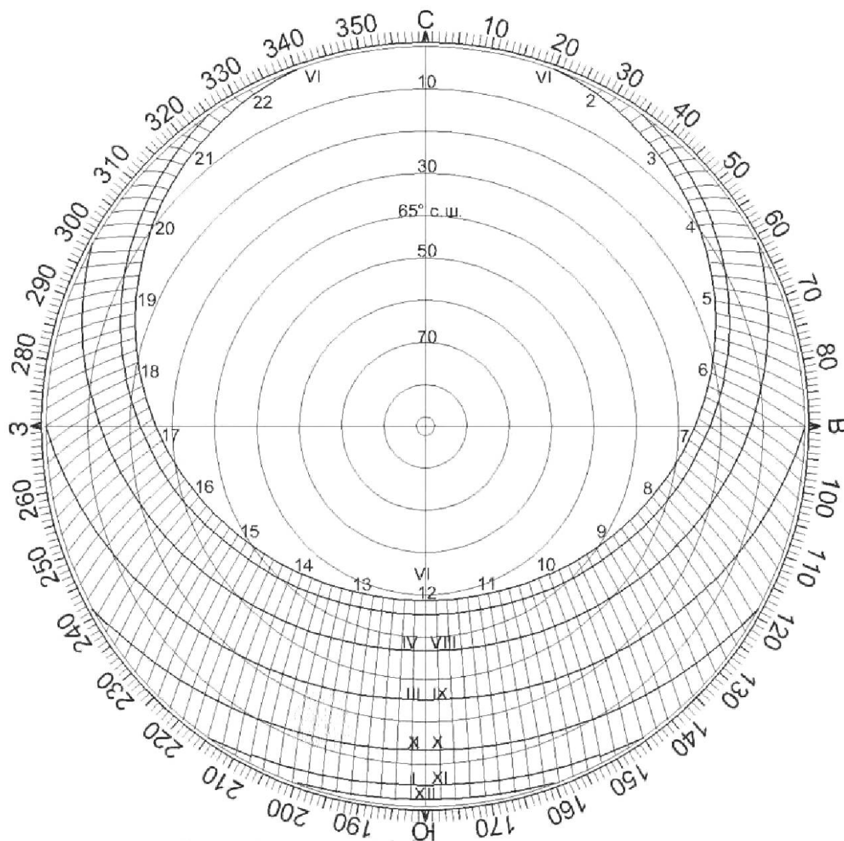
Рисунок Г.10 — Солнечная карта с равнопромежуточными альмукантаратами для территории Российской Федерации, расположенной на 65° с. ш.
