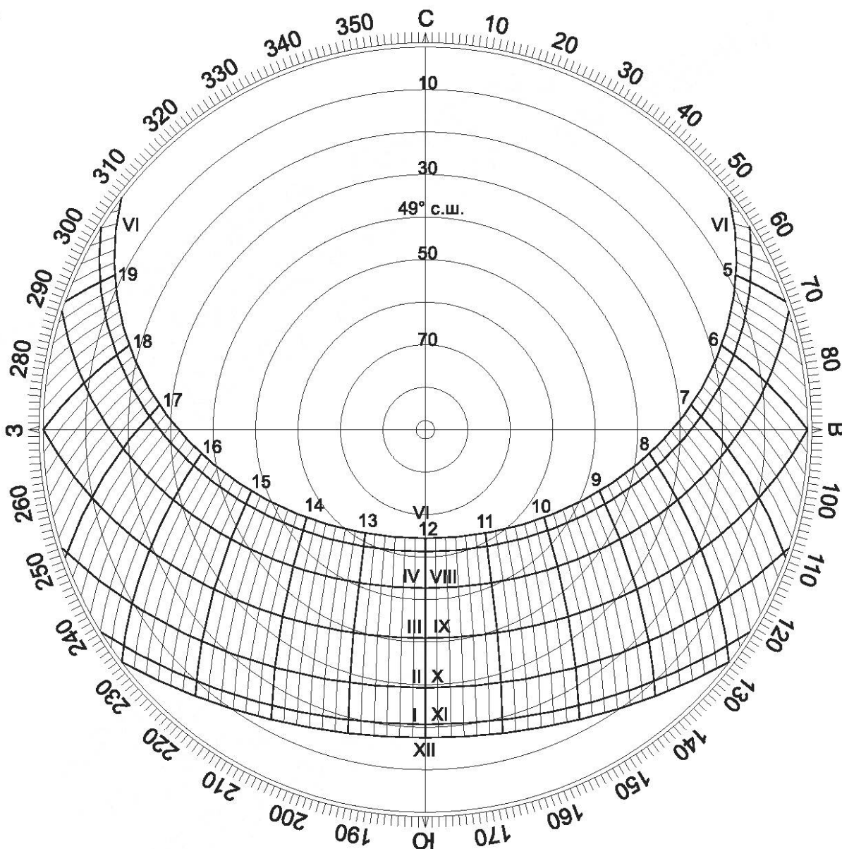
Рисунок Г.5а — Солнечная карта с равнопромежуточными альмукантаратами для территории Российской Федерации, расположенной на 49° с. ш.
