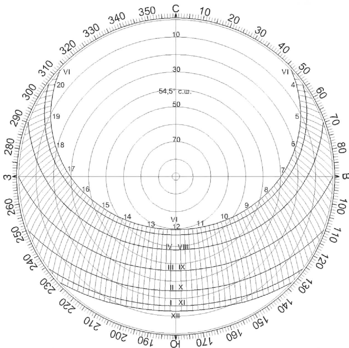
Рисунок Г.12 — Солнечная карта с равнопромежуточными альмукантаратами для города Москвы на 54,5° с. ш.
