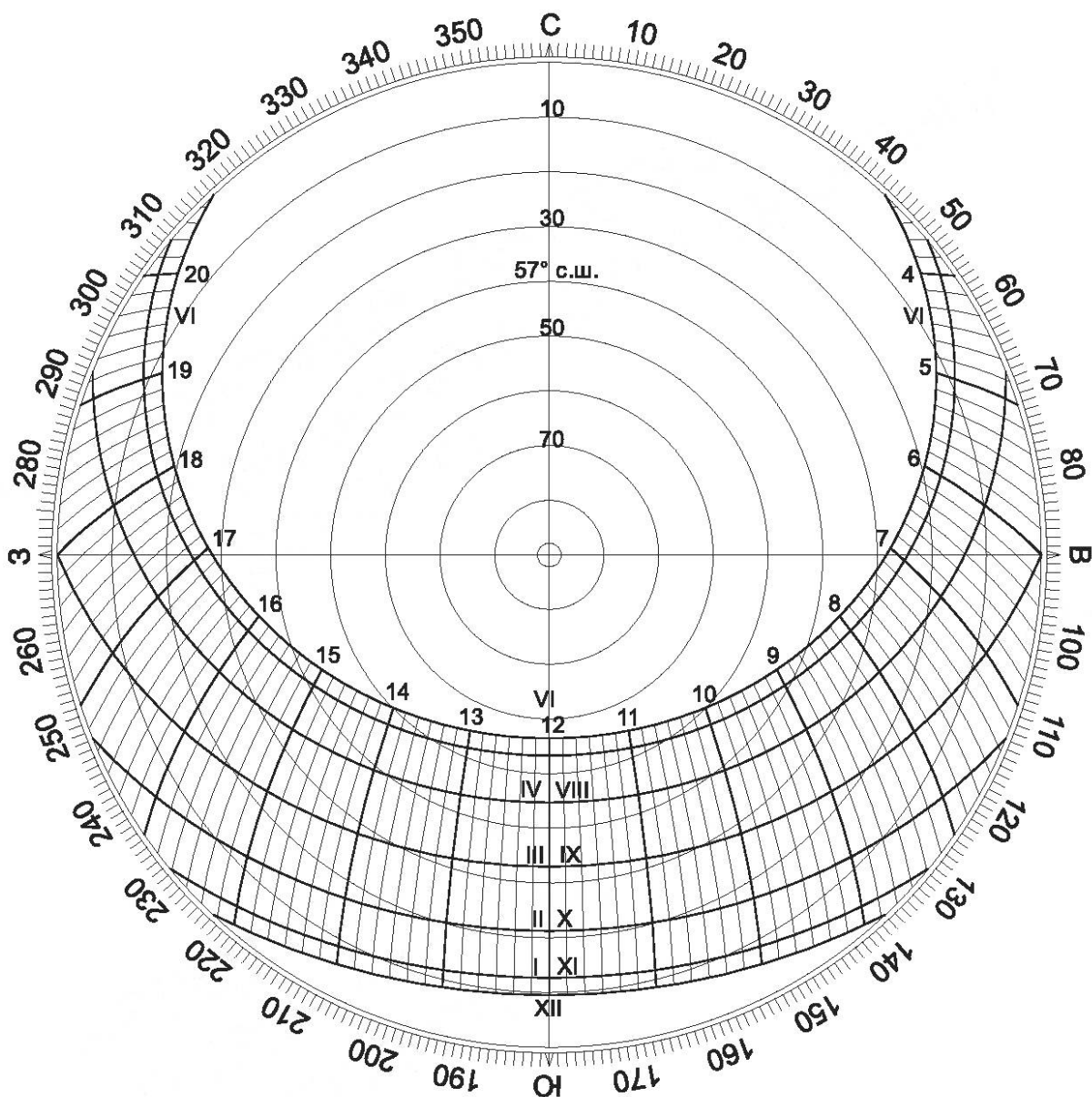
Рисунок Г.6в — Солнечная карта с равнопромежуточными альмукантаратами для территории Российской Федерации, расположенной на 57° с. ш.».
