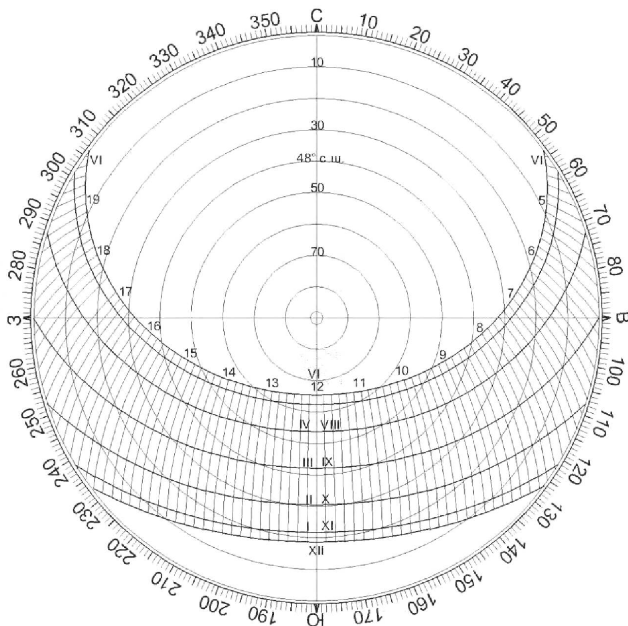
Рисунок Г.5 — Солнечная карта с равнопромежуточными альмукантатами для территории Российской Федерации, расположенной на 48° с. ш.
