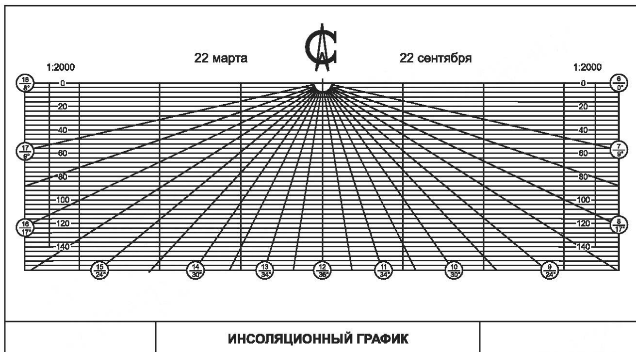
Рисунок 1 — Пример инсоляционного графика, разработанного применительно к дням весеннего (осеннего) равноденствия
