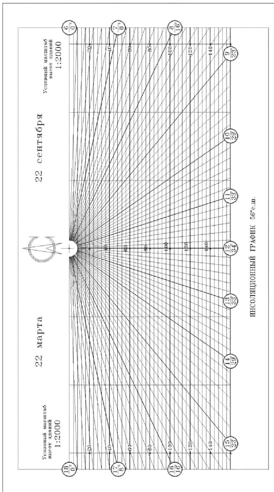
Рисунок В.23 — Инсоляционный график для города Москвы (56° с. ш.) в масштабе 1:2000
