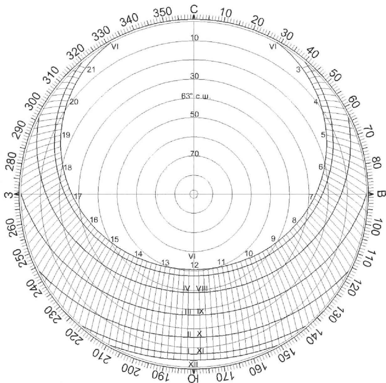
Рисунок Г.9 — Солнечная карта с равнопромежуточными альмукантаратами для территории Российской Федерации, расположенной на 63° с. ш.
