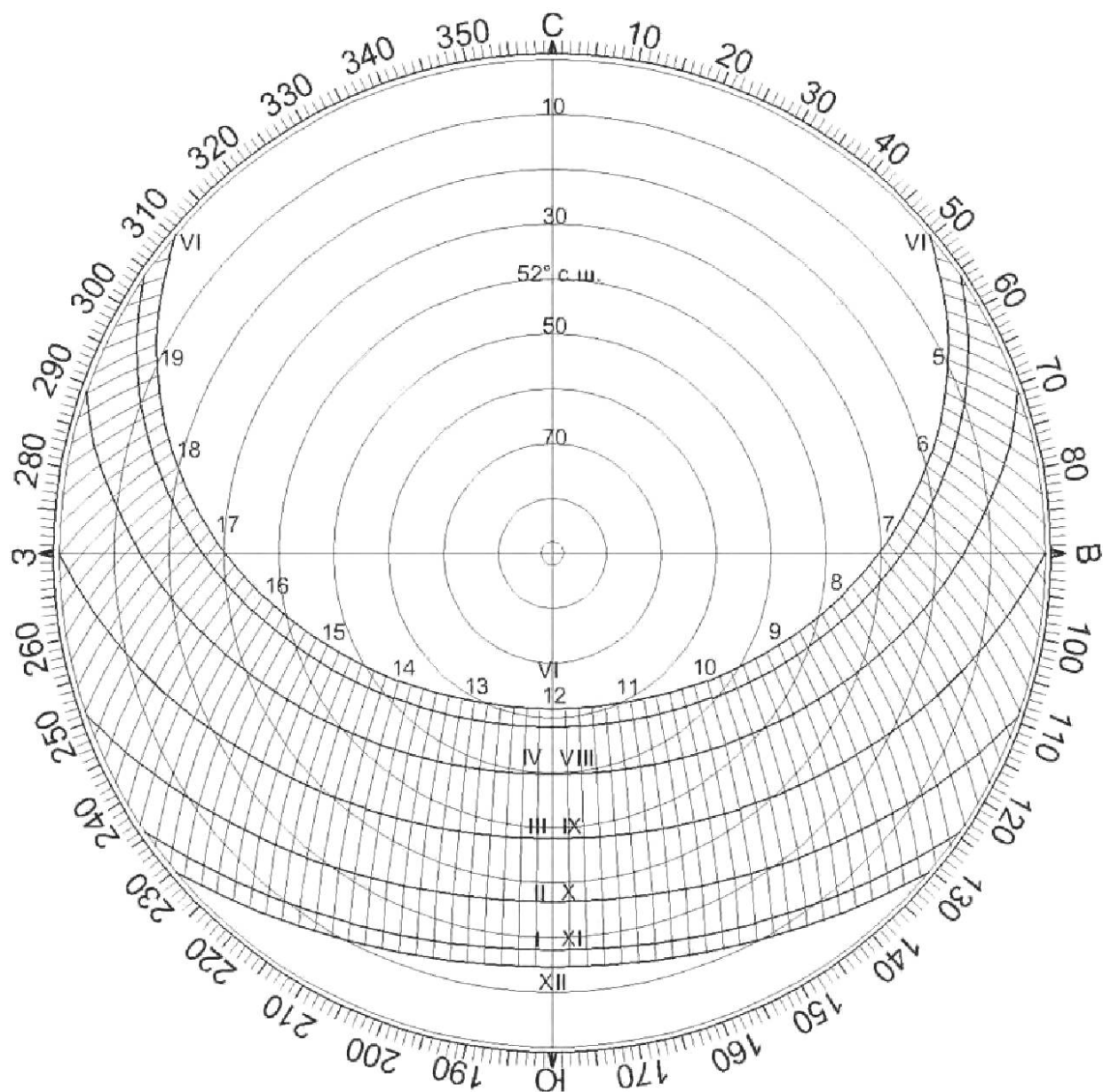
Рисунок Г.6 — Солнечная карта с равнопромежуточными альмукантаратами для территории Российской Федерации, расположенной на 52° с. ш.
