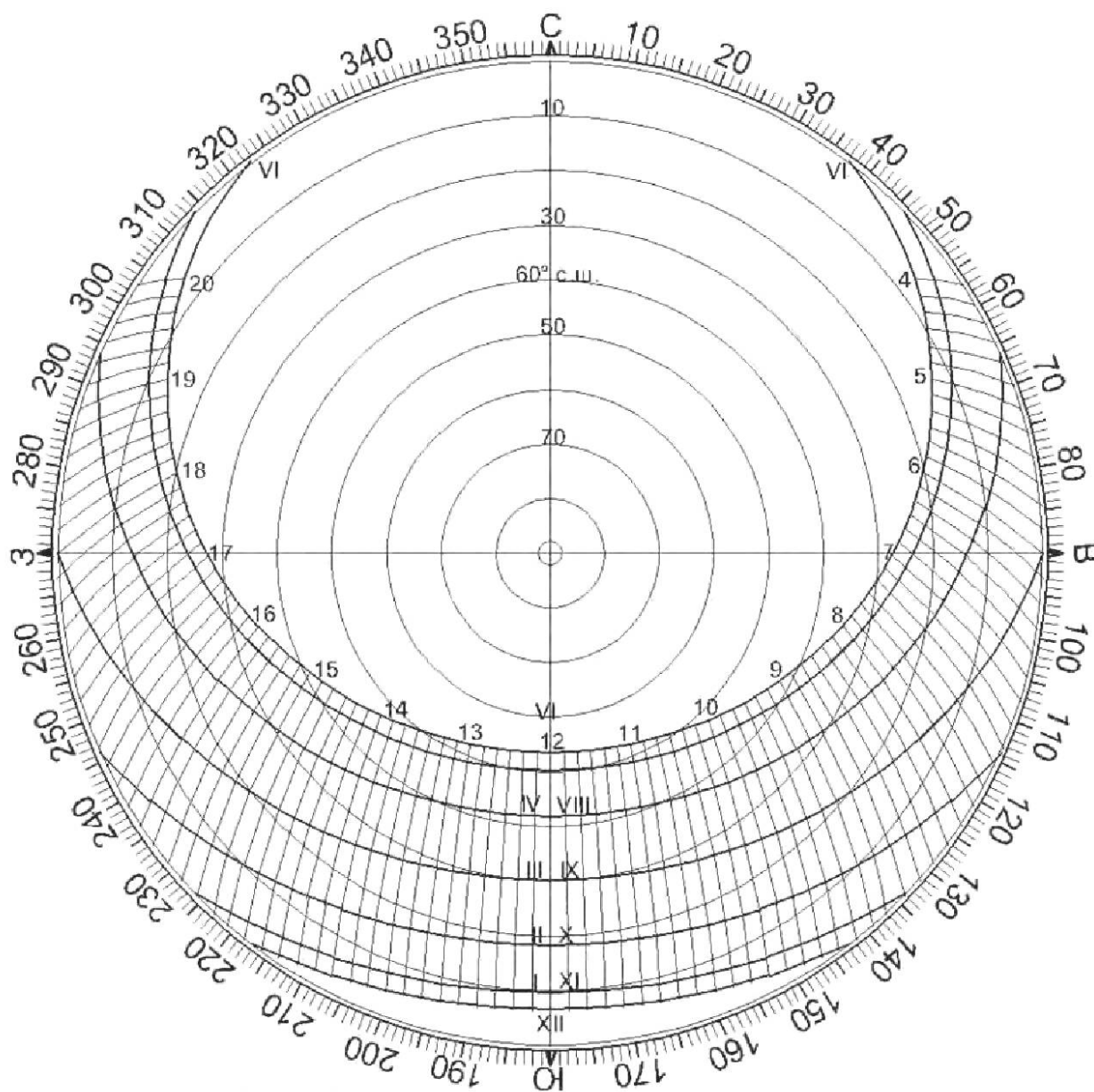
Рисунок Г.8 — Солнечная карта с равнопромежуточными альмукантаратами для территории Российской Федерации, расположенной на 60° с. ш.
