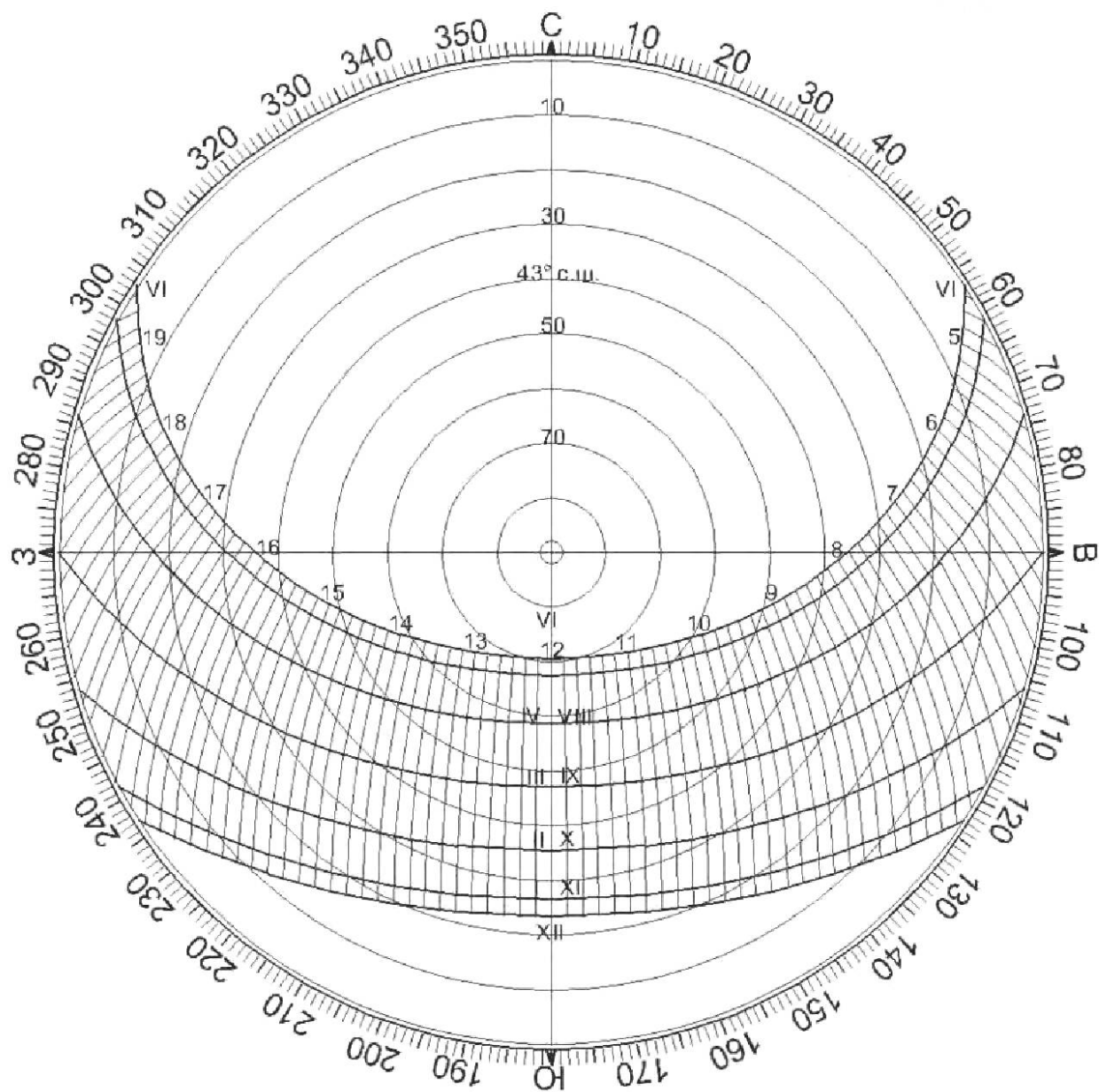
Рисунок Г.2 — Солнечная карта с равнопромежуточными альмукантаратами для территории Российской Федерации, расположенной на 43° с. ш.
