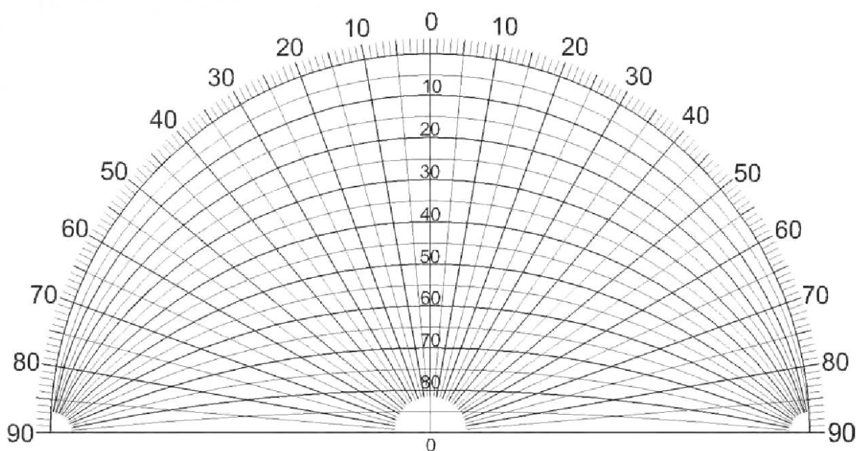
Рисунок Г.1 — Теневой угломер (контурная сетка) для солнечных карт с равнопромежуточными альмукантаратами
