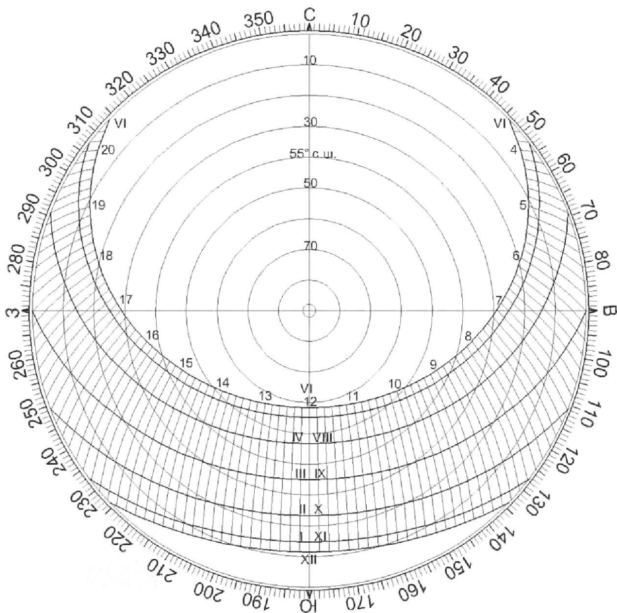
Рисунок Г.13 — Солнечная карта с равнопромежуточными альмукантаратами для города Москвы на 55° с. ш.
