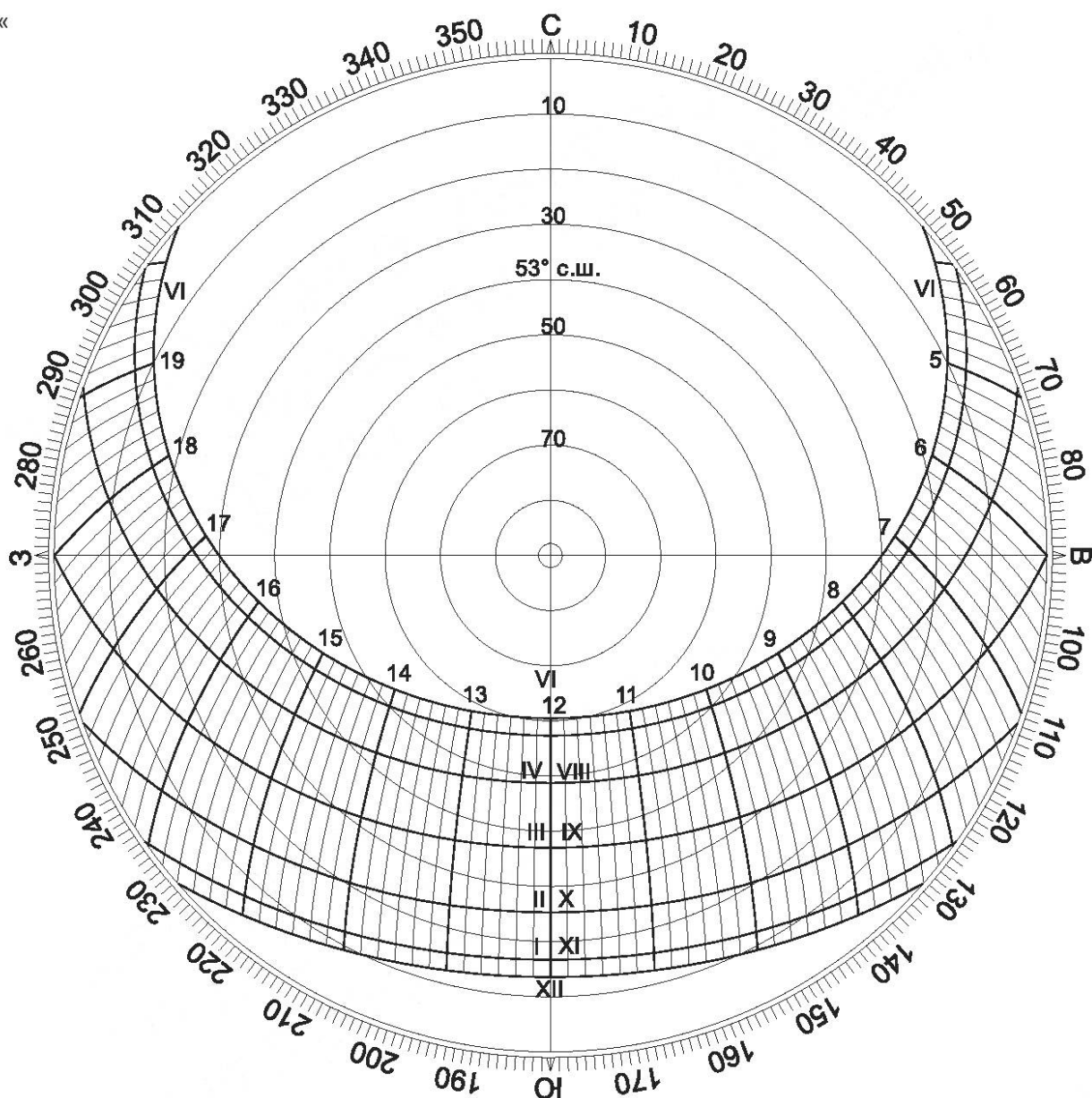
Рисунок Г.6а — Солнечная карта с равнопромежуточными альмукантаратами для территории Российской Федерации, расположенной на 53° с. ш.
