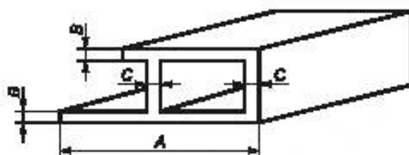
A — размер фальеры; B — толщина стенки открытого профиля; C — толщина стенки закрытого профиля
