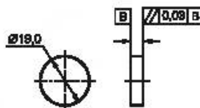
Рисунок 6 — Образец круглого сечения
