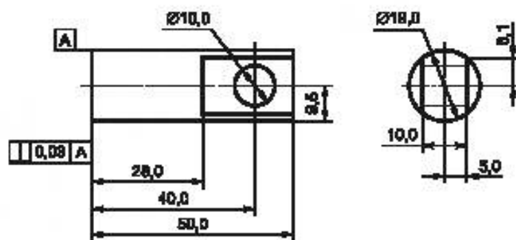
Рисунок 1 — Нагружающий блок, приклеиваемый к образцу круглого сечения
