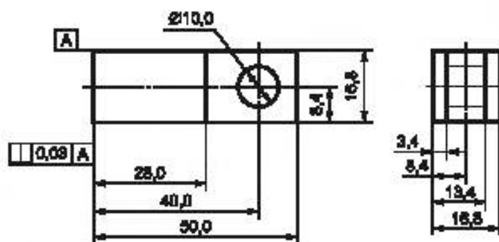
Рисунок 2 — Нагружающий блок, приклеиваемый к образцу квадратного сечения
