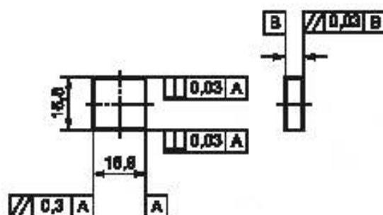
Рисунок 7 — Образец квадратного сечения
