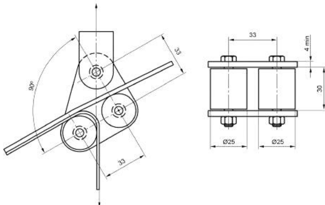
Рисунок 1 — Чертеж приспособления для испытаний
