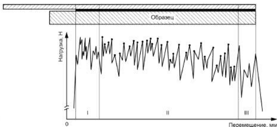
Рисунок 4 — Образец и диаграмма, полученная в ходе испытания
