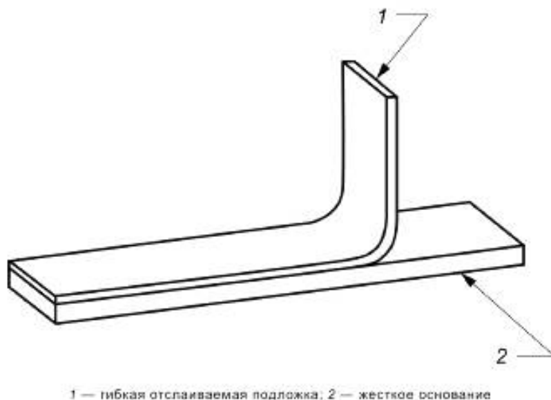
Рисунок 2 — Общий вид образца
