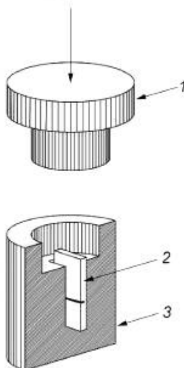
1 — нагружающий поршень; 2 — образец; 3 — корпус с пазом
