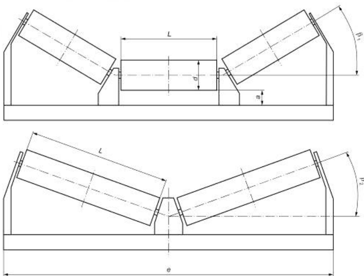
Рисунок 1 — Виды роликоопор
