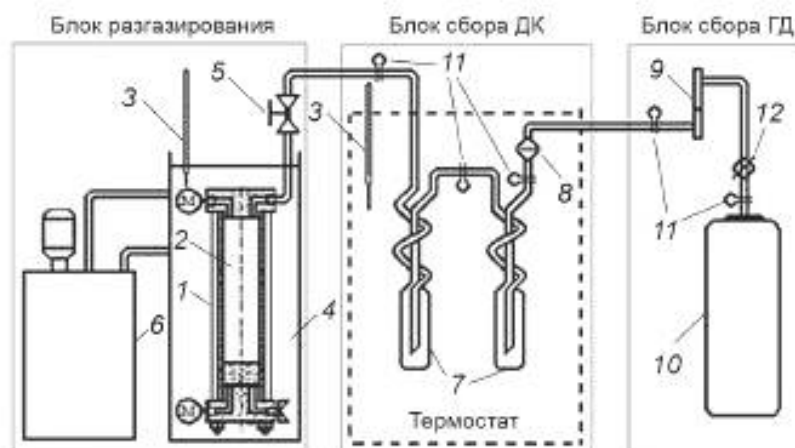
1 — пробоотборник с пробой НГК; 2 — камера с пробой НГК; 3 — термометр; 4 — термостатируемая баня; 5 — вентиль тонкой регулировки; 6 — термостат; 7 — ловушки-приемники дегазированного конденсата; 8 — фильтр; 9 — лабораторный расходомер; 10 — приемник газа дегазации; 11 — заглушки; 12 — трехходовой кран
