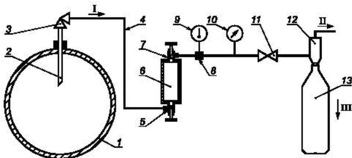
1 — конденсатопровод; 2 — пробоотборное устройство; 3 — запорный вентиль конденсатопровода; 4 — пробоотборная линия; 5, 7 — вентили пробоотборника; 6 — пробоотборник; 8 — карман для термометра; 9 — термометр; 10 — манометр; 11 — вентиль; 12 — сепаратор; 13 — емкость для сбора жидкости. Материальные потоки: I — НГК, II — газ дегазации НГК на сброс, III — жидкий остаток дегазации НГК
