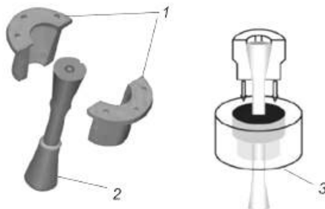
1 — разъемная зажимная втулка с конусным внутренним стержнем; 2 — образец; 3 — опора
