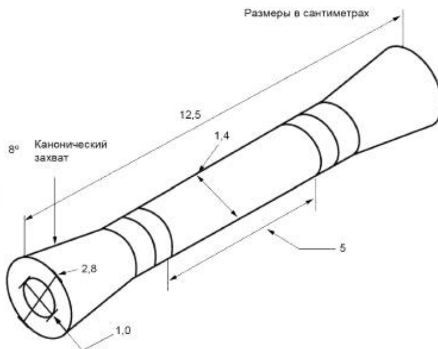
Рисунок В.4 — Образец с коническими захватными участками
