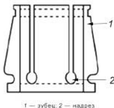
Рисунок А.3 — Зажимная втулка
