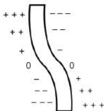
S-образный изгиб
