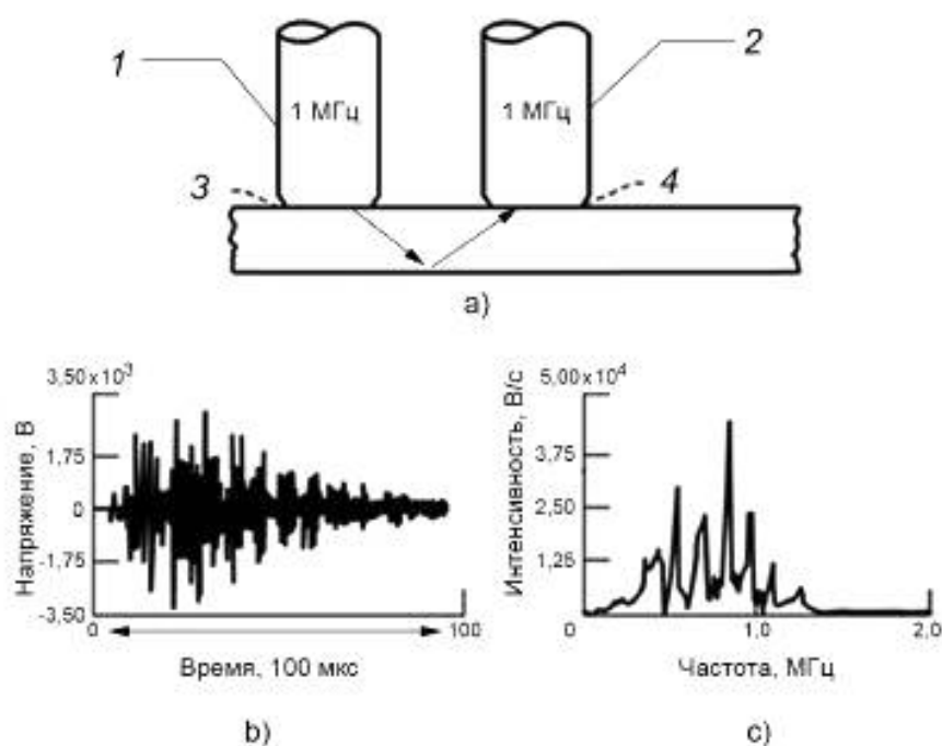
а) — датчики лоперечной передачи; б) — форма волны множественных отклонений; в) — спектр переданной формы волны
